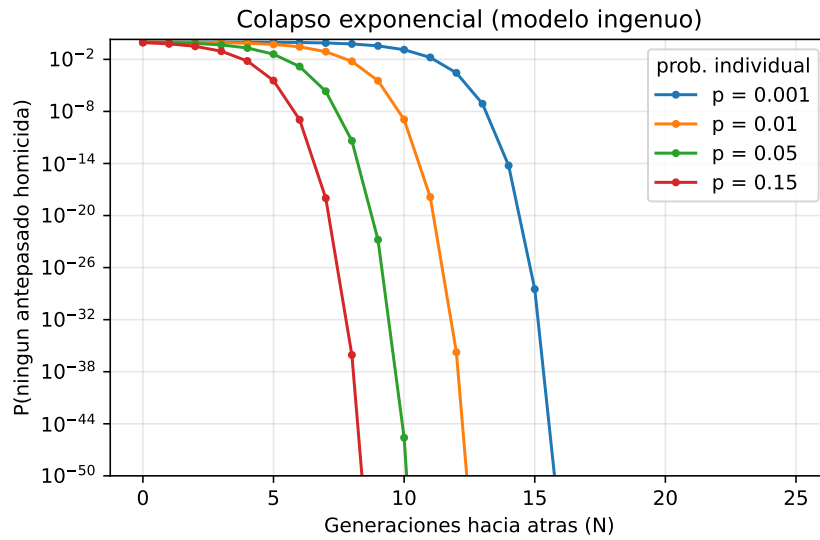
Figura 1: Colapso exponencial de P_{\text{ing}}(p, N) (escala logarítmica) según el modelo ingenuo, Ec. (2).
