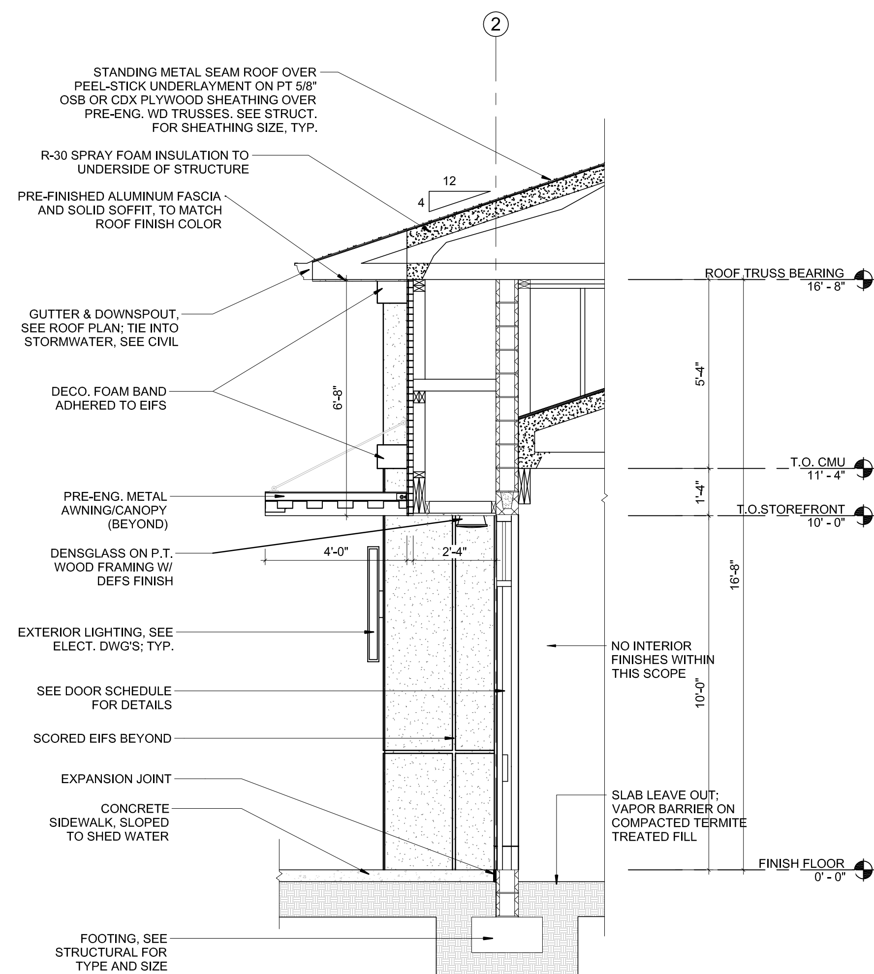
SCALE: 1/4"=1'-0" 21
