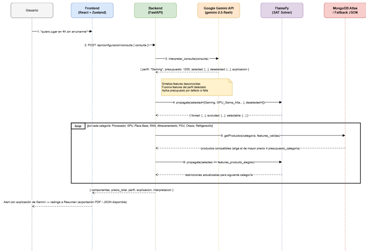
Ilustración 13: Diagrama de secuencia (consulta en lenguaje natural)
