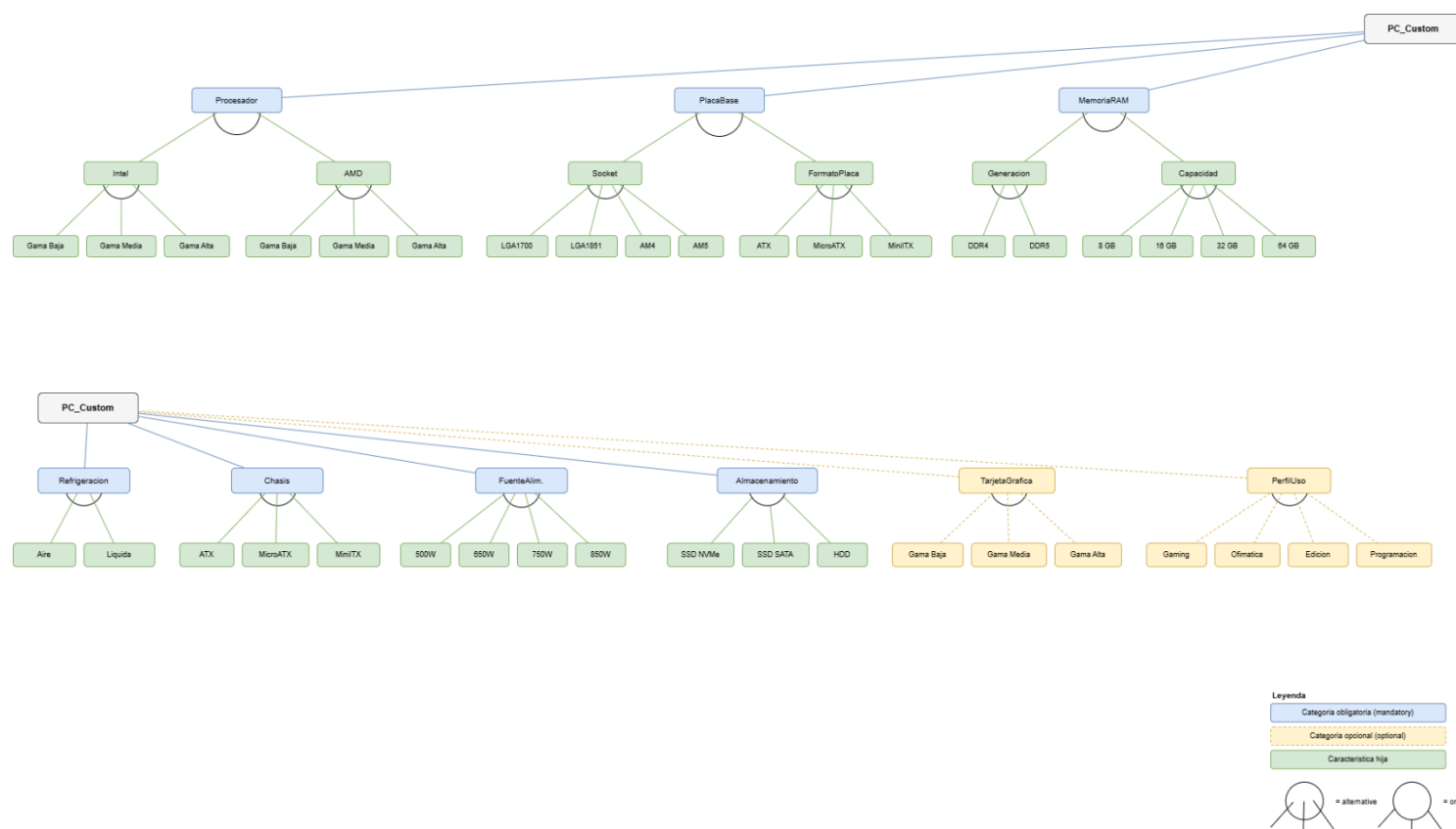
Ilustración 15: Modelo de características (representación visual)
