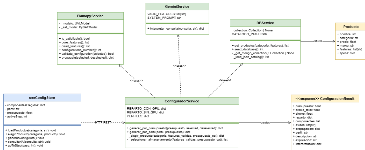
Ilustración 12: Diagrama de clases
