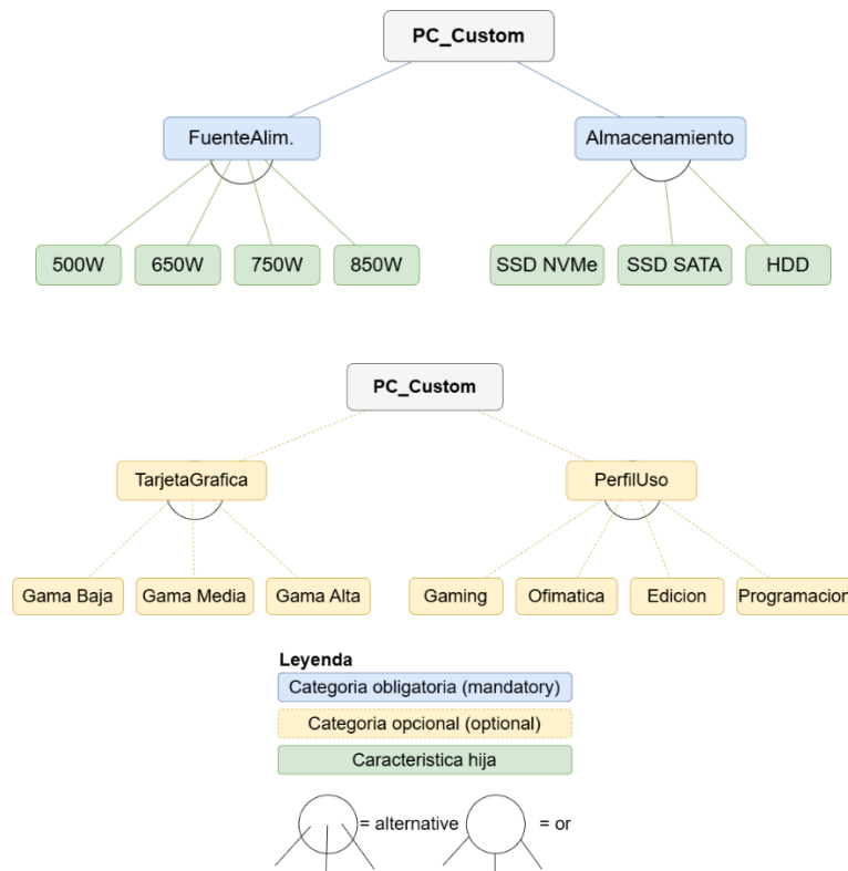
Ilustración 16: Modelo de características (representación visual)
