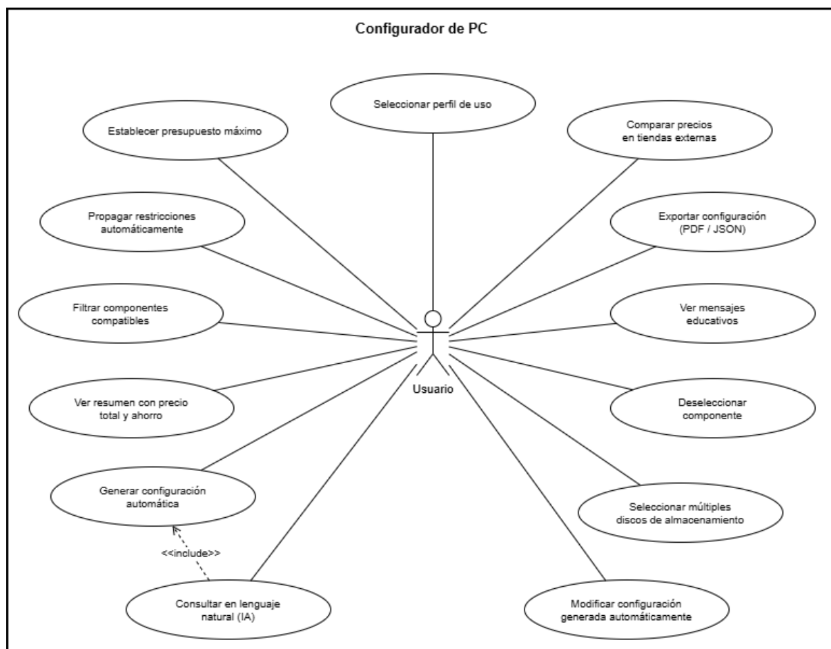
Ilustración 10: Casos de uso
