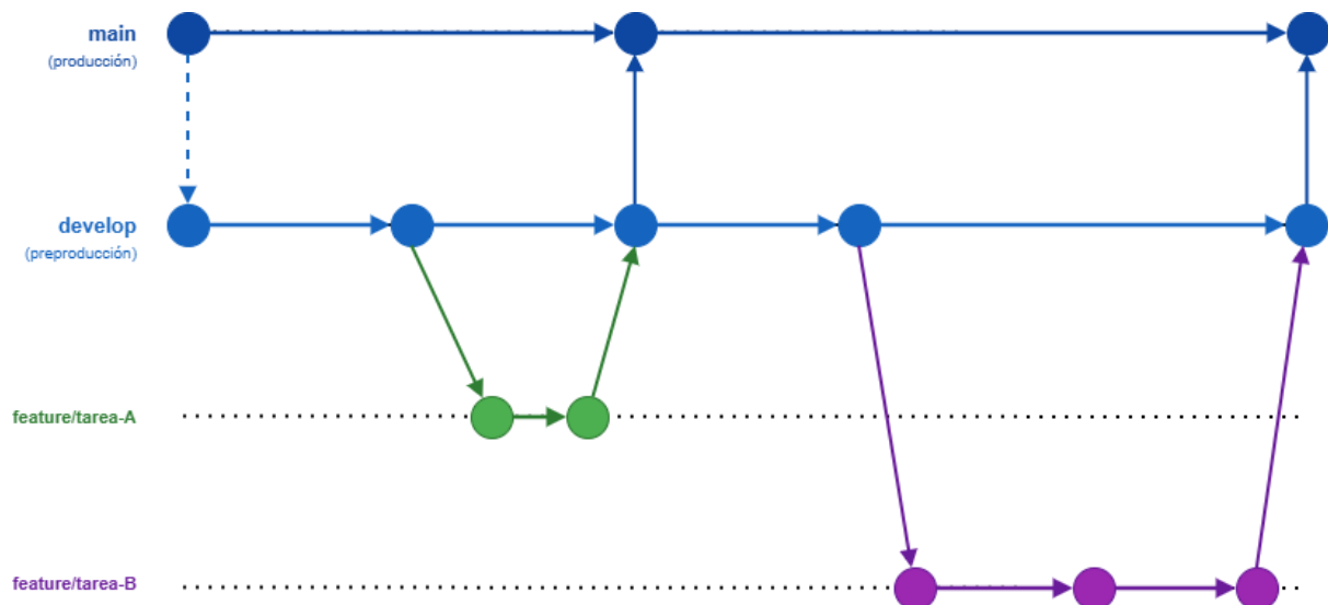
Ilustración 26: Estrategia de ramas
