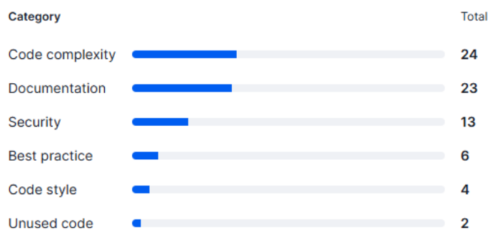
Ilustración 29: Número de issues detectados
