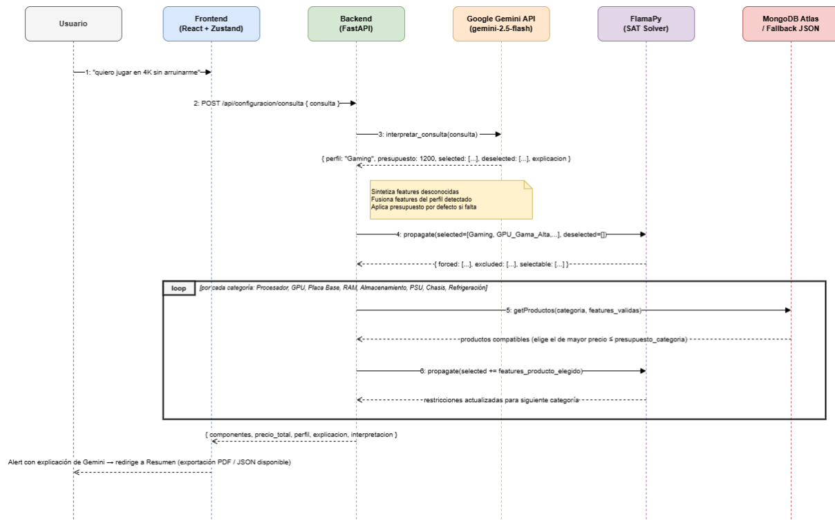
Ilustración 13: Diagrama de secuencia (consulta en lenguaje natural)
