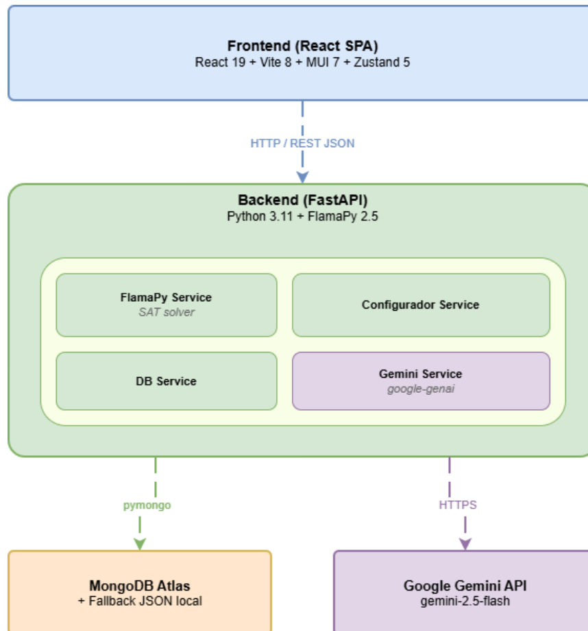
Ilustración 11: Arquitectura del sistema
