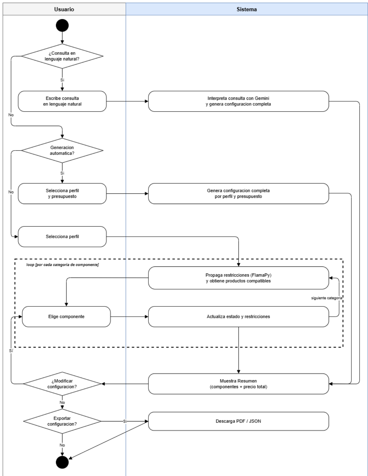
Ilustración 14: Diagrama de actividades
