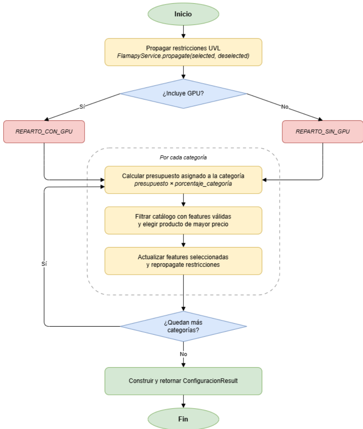
Ilustración 16: Diagrama de flujo del algoritmo generar_por_presupuesto()
