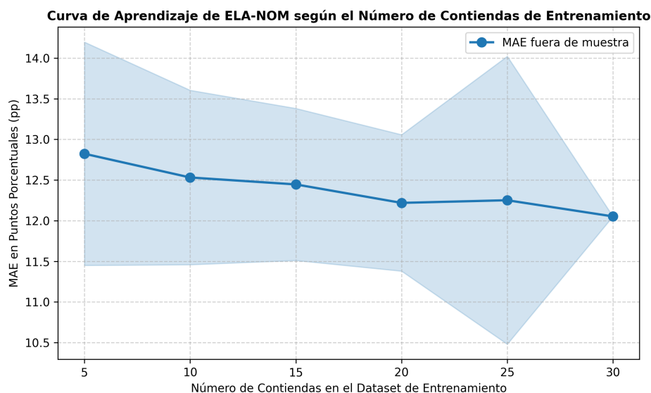
Figura 6.7: Curva de aprendizaje de ELA-NOM. MAE fuera de muestra (media y banda \pm 1 desviación estándar) en función del número de contiendas de entrenamiento. La banda sombreada representa la variabilidad entre las 50 repeticiones de muestreo.
