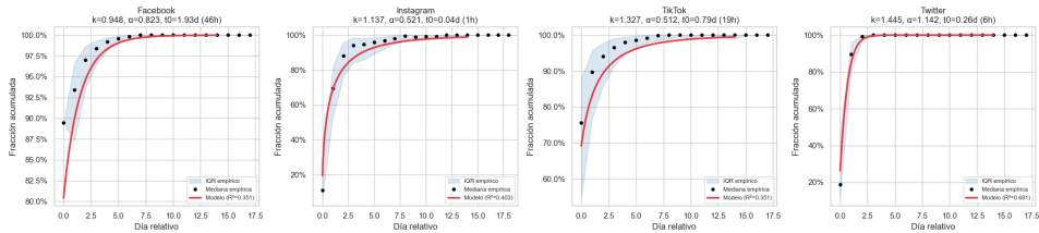
Modelos Weibull con offset por plataforma
