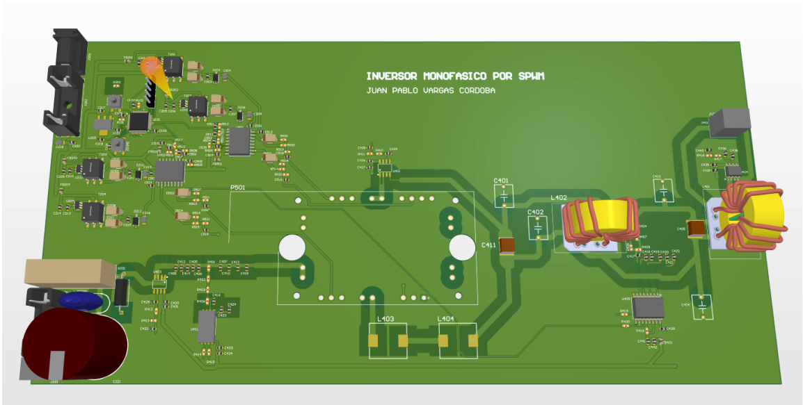
Figura 5: Primera versión del diseño de la PCB del inversor.
