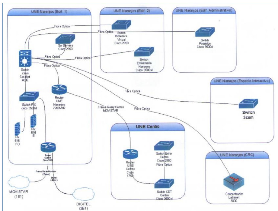
Figura Nro. 1 Diseño Físico y Lógico de la Red
