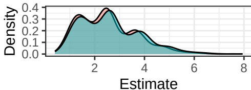
Binomial n = 20
