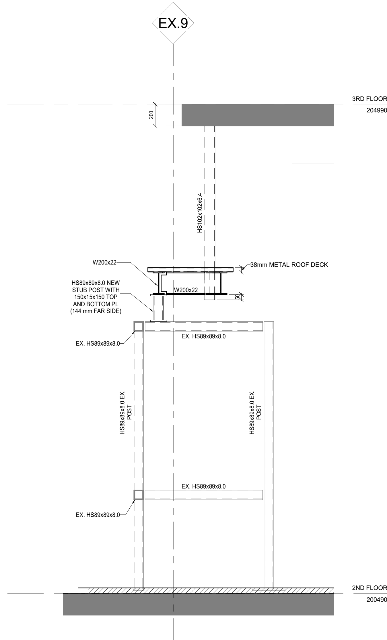
3 SECTION S401/ 1:20
