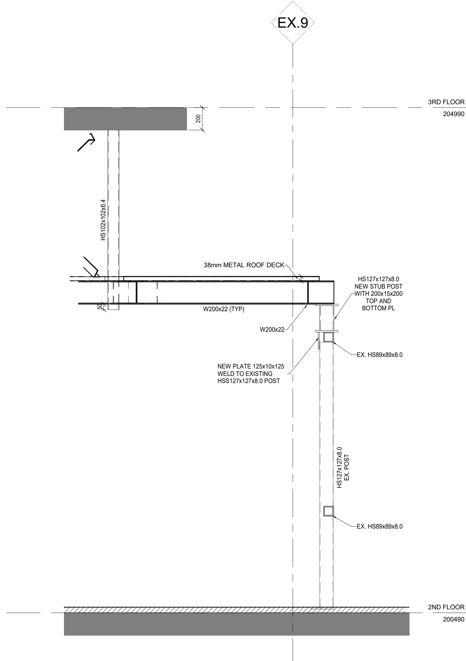
2 SECTION S401/ 1:20
