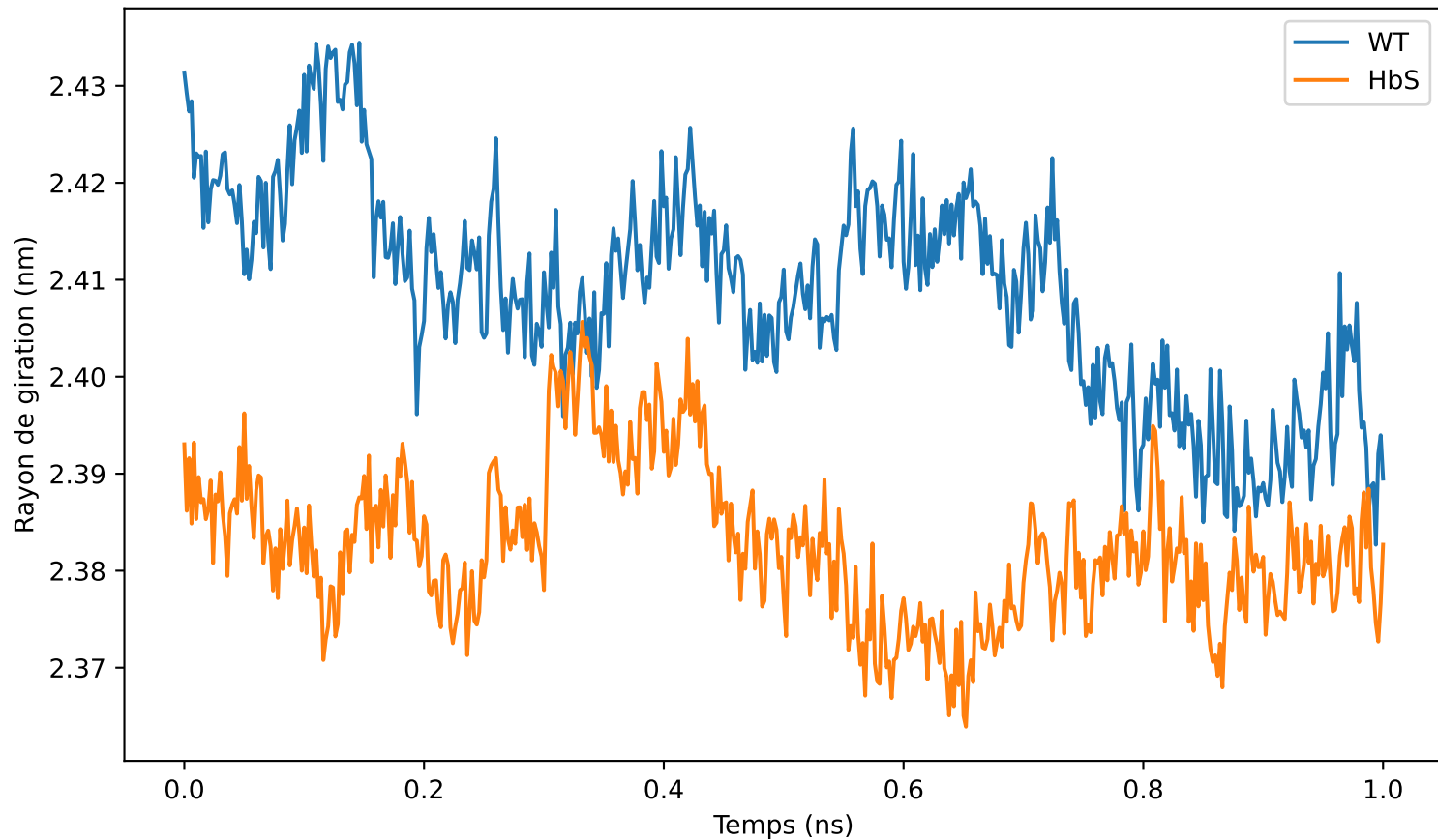
Compacité structurale : WT vs HbS
