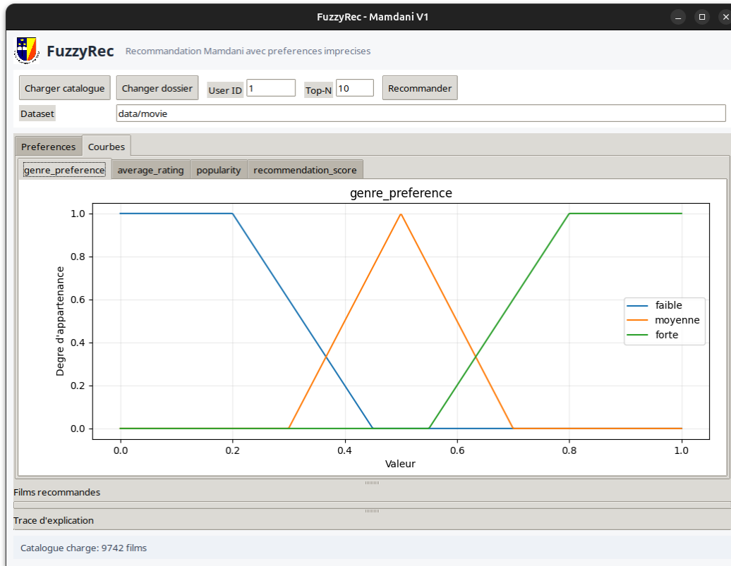
FIGURE 9 – Onglet des courbes : les fonctions d'appartenance des variables linguistiques sont integrees dans la GUI afin de rendre visible la transformation des preferences.
