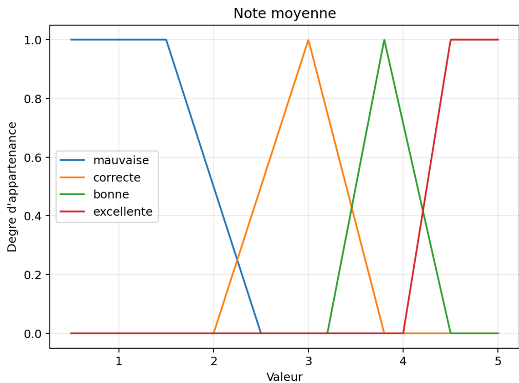
FIGURE 3 – Fonctions d'appartenance de la note moyenne.
