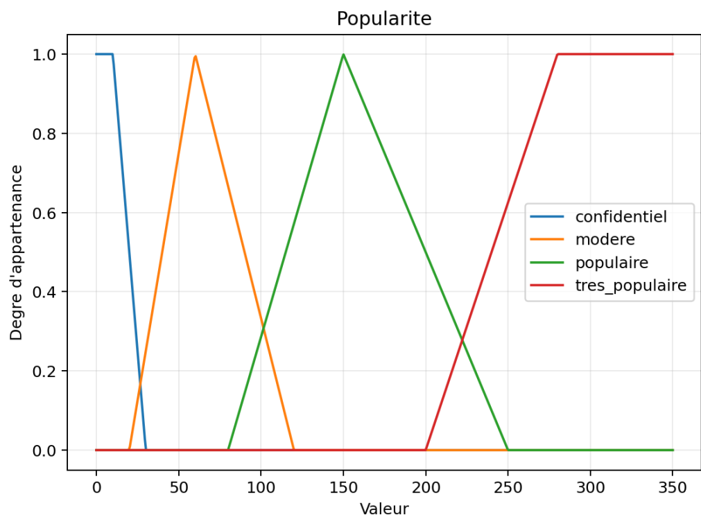
FIGURE 4 – Fonctions d'appartenance de la popularite.
