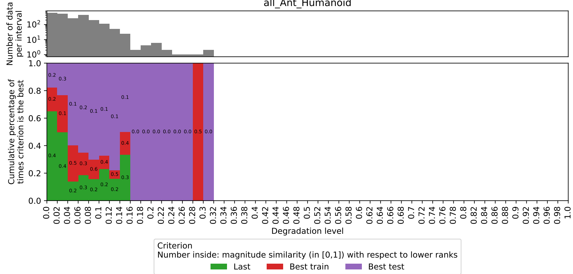
all_Ant_Humanoid
