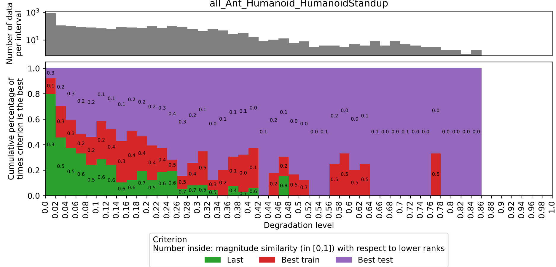
all_Ant_Humanoid_HumanoidStandup
