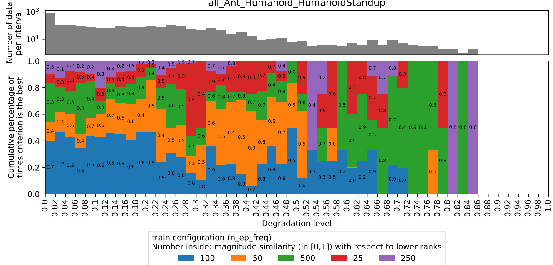
all_Ant_Humanoid_HumanoidStandup
