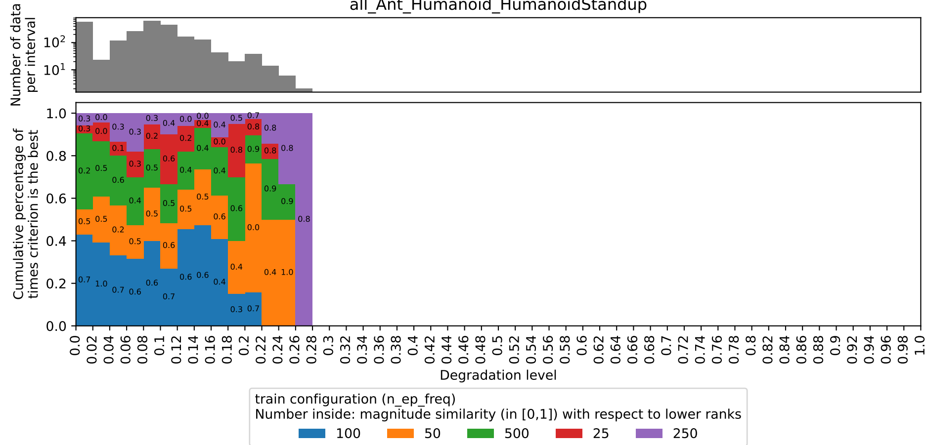
all_Ant_Humanoid_HumanoidStandup
