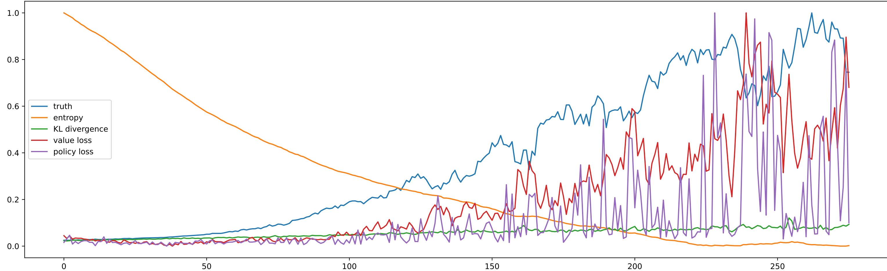
PPO_Ant_seed1
