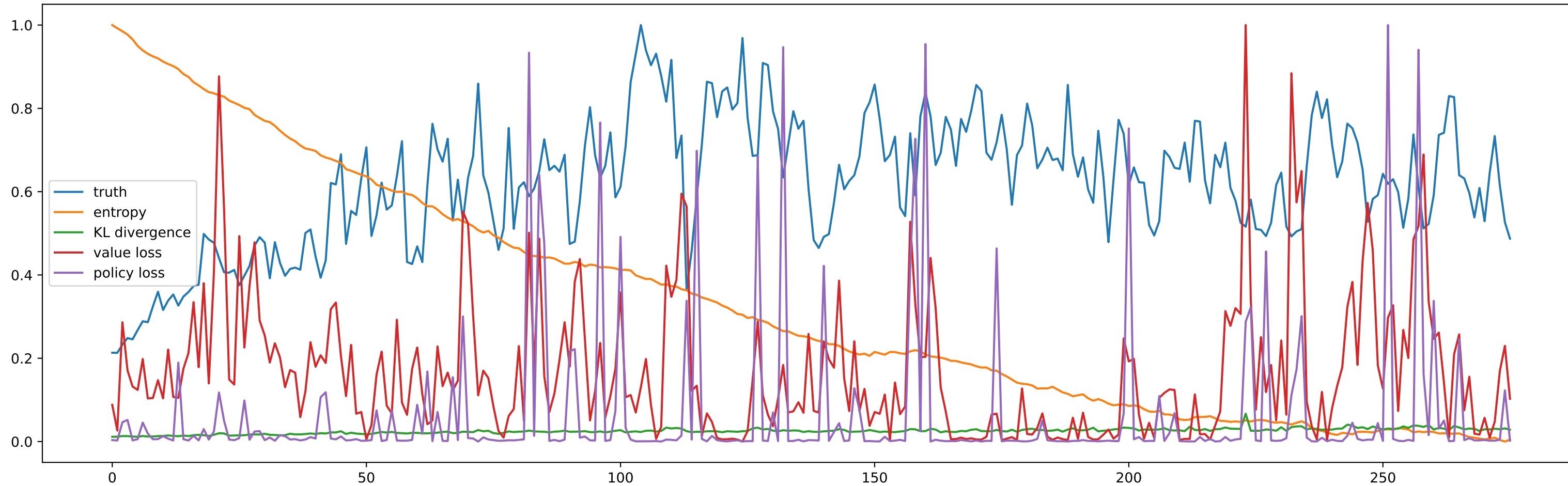
PPO_Hopper_seed2
