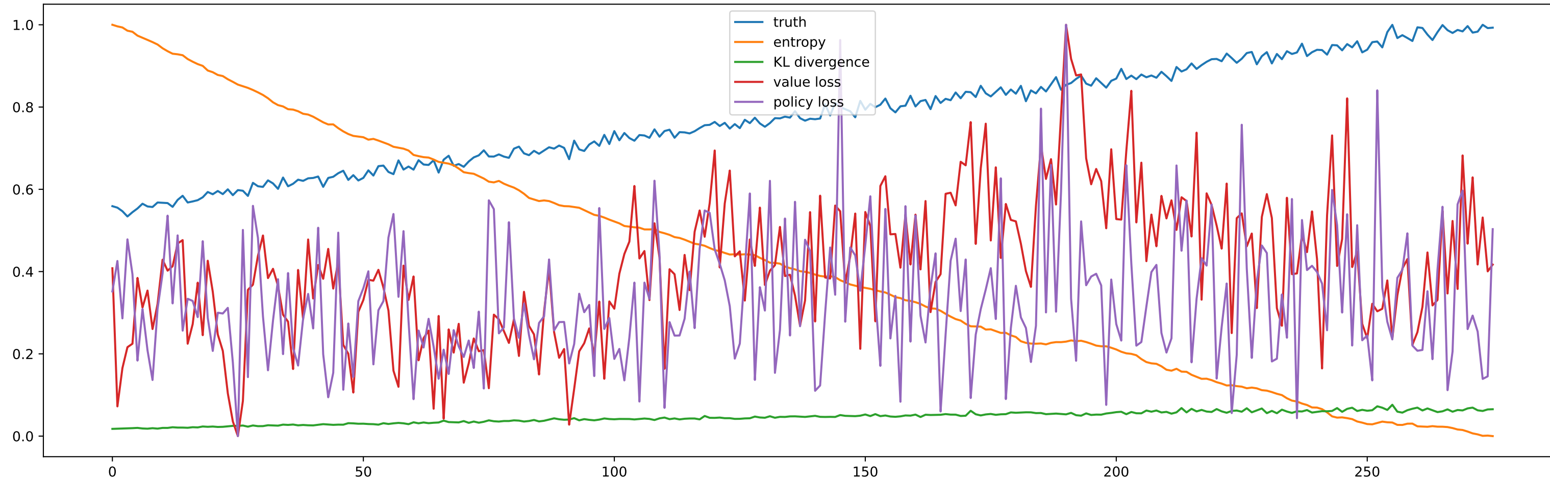
PPO_Humanoid_seed1
