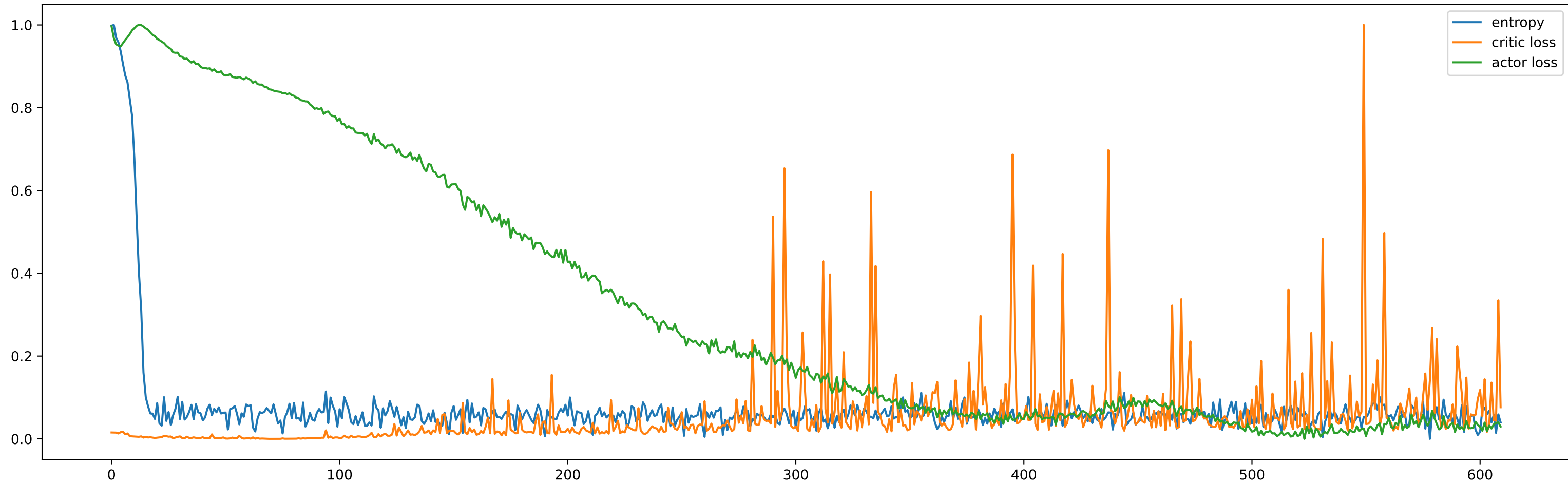
SAC_Ant_seed1
