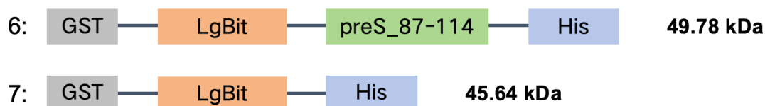
图 3-17 构建不含 foldon 三聚化结构域的 GST-LgBiT-preS 87-114-His 和 GST-LgBiT-His。
