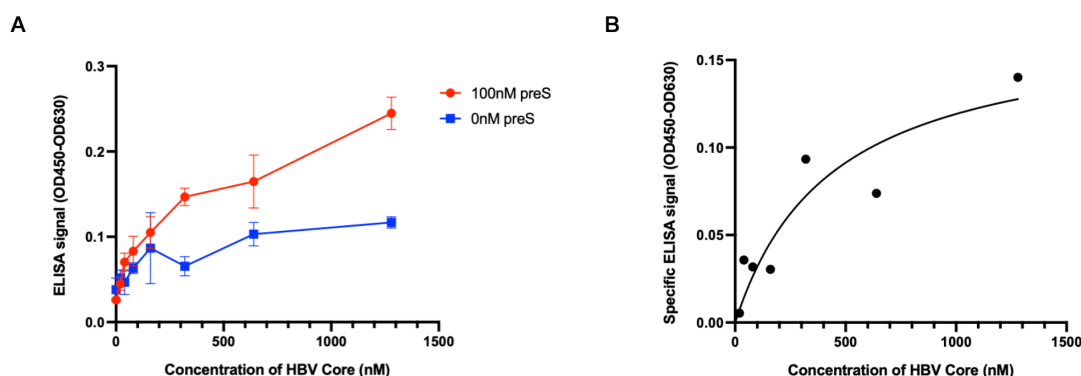
图 3-6 替换抗 HBc IgG D4 后的 StrepXT 捕获 preS ELISA 结果。A，100 nM 和 0 nM preS 包被后 HBc 的滴定曲线，误差线表示重复孔标准差。B，HBc 滴定的特异性信号。中高浓度 HBVCp149 条件下信噪比有所增加，但 Z-factor 仍未达到稳健筛选所需水平。
