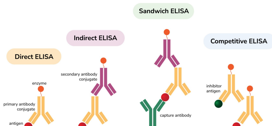
图 2-1 四种 ELISA 类型示意图。直接 ELISA、间接 ELISA、夹心 ELISA 和竞争 ELISA 采用不同的抗原固定、抗体识别和酶标检测方式，将抗原-抗体结合转换为酶促信号。图片来源 vecteezy。
