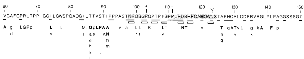
图 1-3 preS 功能区的序列保守性。图中比较 32 个 HBV 分离株，并以灰色区域标示 Asn98-Ser124 附近的保守片段；该片段的保守性与连接子替换突变和双丙氨酸突变实验中的病毒颗粒形成表型一致，引自文献 [20] 。
