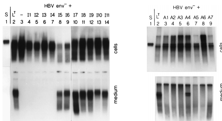
图 1-2 preS 短线性区域对 HBV 感染性病毒颗粒形成的重要性。左图显示连接子替换实验：I1-I14 突变体不能恢复缺失 L 蛋白表达的 HBV 基因组的感染性病毒颗粒分泌，而 I5-I11 突变体可以恢复分泌。右图显示双丙氨酸扫描实验：A1-A3 和 A5-A7 突变体削弱或阻断感染性病毒颗粒形成，而突变非保守残基的 A4 仍保留感染性病毒颗粒形成能力，引自文献 [20] 。
