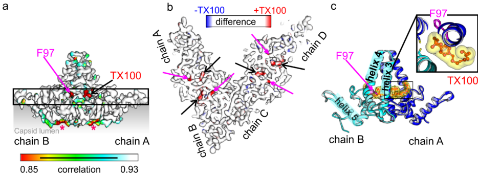
图 1-4 Triton X-100 相关密度位于 HBc 二聚体界面附近，与 F97 等局部构象变化相关，引自文献 [25] 。
