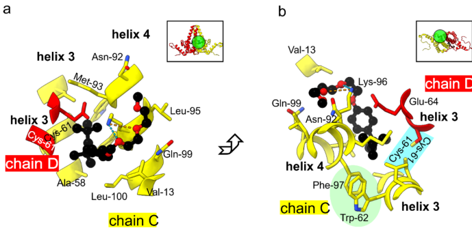
图 1-5 Triton X-100 被链 C 和链 D 形成的特定口袋容纳，引自文献 [25] 。
