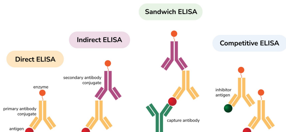
图 2-1 四种 ELISA 类型示意。直接、间接、夹心和竞争 ELISA 在抗原固定、抗体识别和酶标读出方式上不同，均把抗原-抗体结合转换为酶促信号。图片来源：Vecteezy [32] 。
