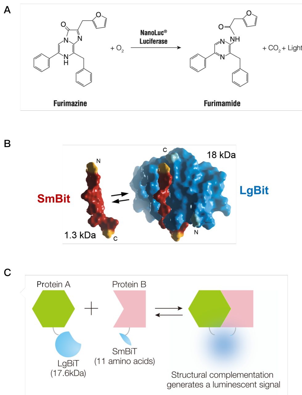
图 2-3 NanoLuc 与 NanoBiT 蛋白互补技术原理。A，NanoLuc 催化 furimazine 氧化并产生发光信号。B，NanoBiT 由 SmBiT 和 LgBiT 组成，二者互补后恢复 NanoLuc 活性。C，SmBiT 和 LgBiT 分别融合到两个待测蛋白上时，目标蛋白靠近可带来发光信号，引自文献 [33] 。
