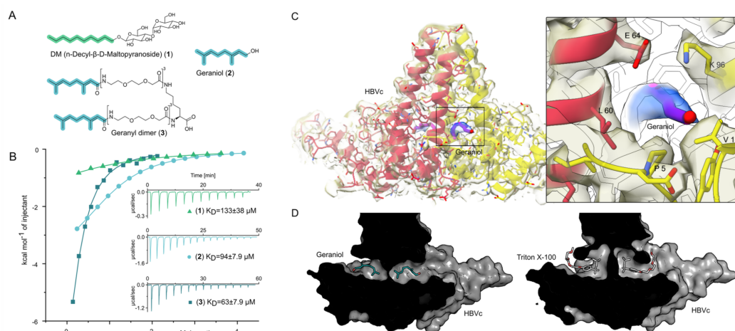
图 1-6 香叶醇结合 HBc 中心疏水口袋及其与 Triton X-100 结合位点的比较。化学结构、ITC 结合曲线、冷冻电镜密度和口袋剖面显示，香叶醇可与 HBc 核心蛋白相互作用，并结合在可容纳疏水分子的特定口袋中；同一研究还分析了香叶基二聚体对该口袋的结合，引自文献 [26] 。
