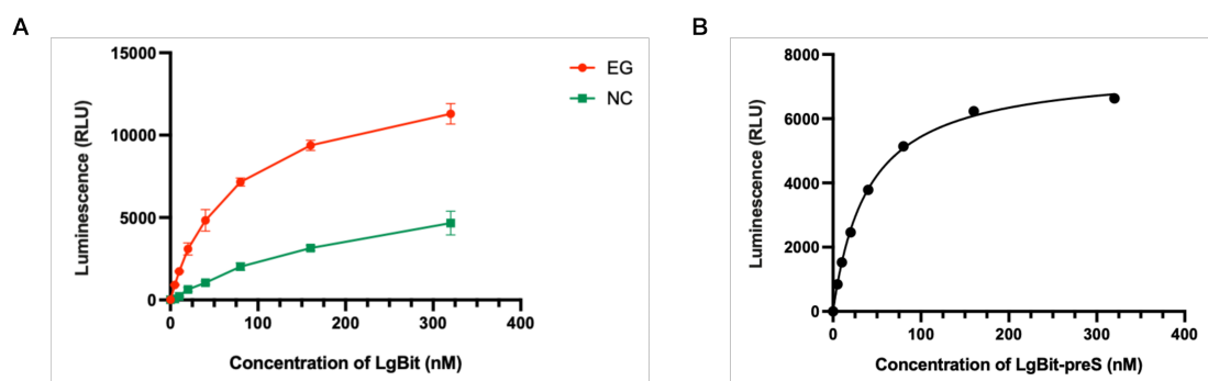
图 3-14 固定 HBVCp182-SmBiT 浓度为 12.5 nM 后滴定含 preS 87-114 的 LgBiT 融合蛋白。A，实验组信号随 LgBiT-preS 浓度升高而增加，误差线表示同一实验内重复孔的 SD。B，扣除阴性对照后的特异性信号呈饱和趋势；Langmuir 单一位点吸附模型拟合得到当前 NanoBiT 构型下的表观参数 K_{app} 约为 39.86 nM，该值不等于热力学 K_D 。
