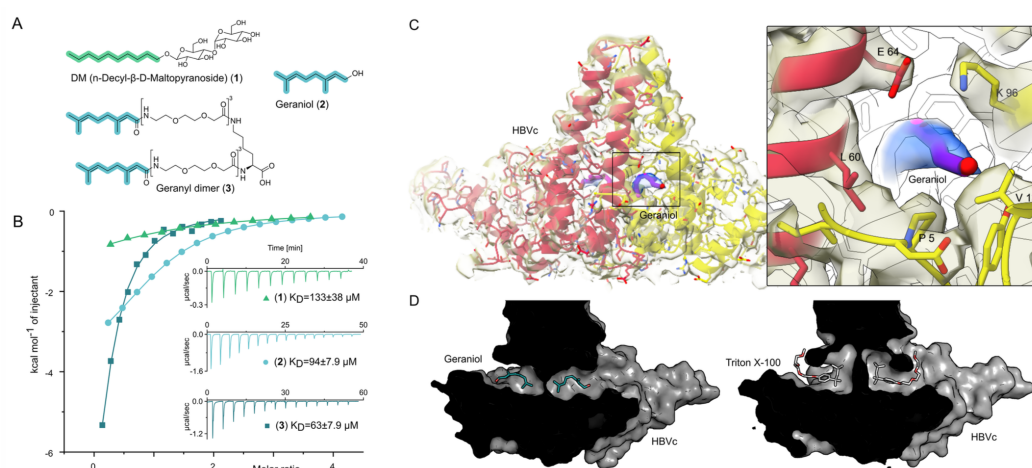
图 1-6 香叶醇结合 HBc 中心疏水口袋及其与 Triton X-100 结合位点的比较。化学结构、ITC 结合曲线、冷冻电镜密度和口袋剖面显示，香叶醇可与 HBc 核心蛋白相互作用，并结合在可容纳疏水分子的特定口袋中；同一研究还分析了香叶基二聚体对该口袋的结合，引自文献 [35] 。
