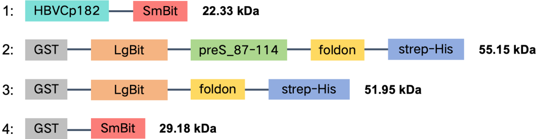
图 3-8 NanoBiT 相关融合蛋白的构建。图中示意 HBVCp182-SmBiT、含 preS 87-114 的 GST-LgBiT-preS、GST-LgBiT 阴性对照和 GST-SmBiT 阳性对照等构建体，用于后续发光互补检测。
