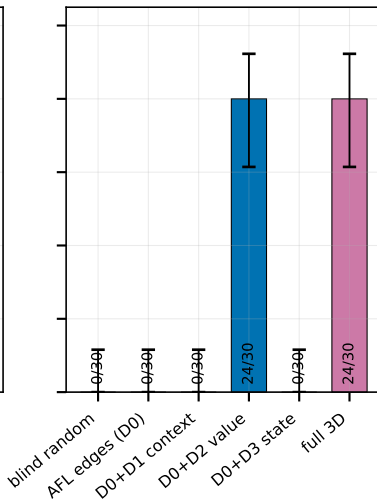
T2_value_range (budget 300,000 execs)
