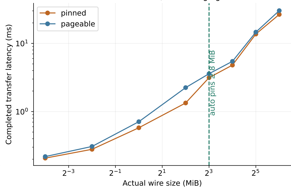
D2H: retained, warm staging
