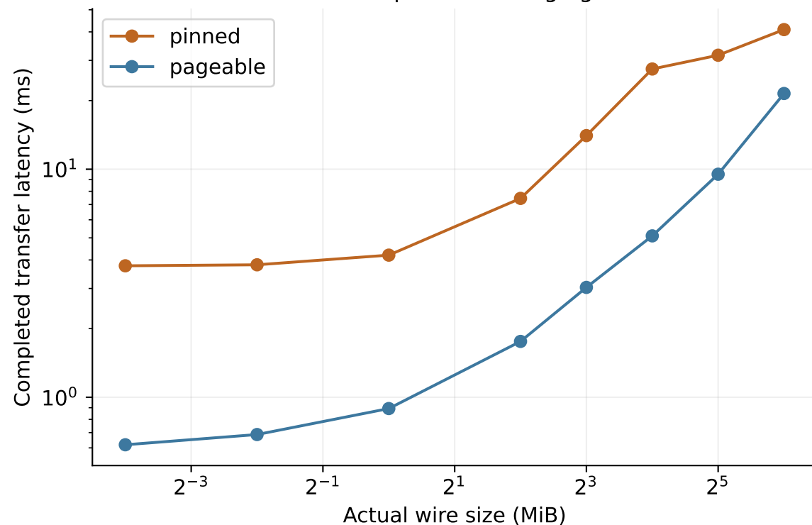
D2H: ephemeral staging
