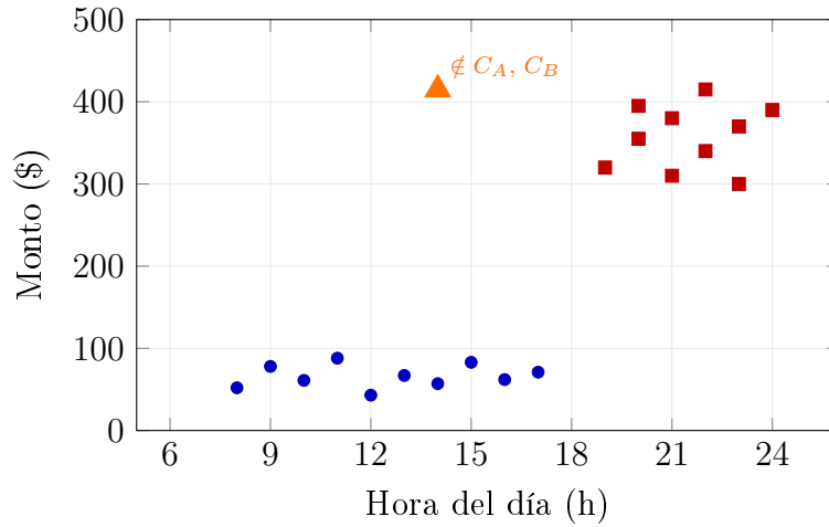
Figura 5: Flujo de transacciones bancarias procesadas por BIRCH. Los clusters C_A (diurno, monto bajo) y C_B (nocturno, monto alto) representan el conocimiento incremental acumulado. La nueva observación (14 h, $415) no supera el umbral de similitud T con ninguno de los dos perfiles existentes, por lo que BIRCH crea un tercer nodo CF [14].
