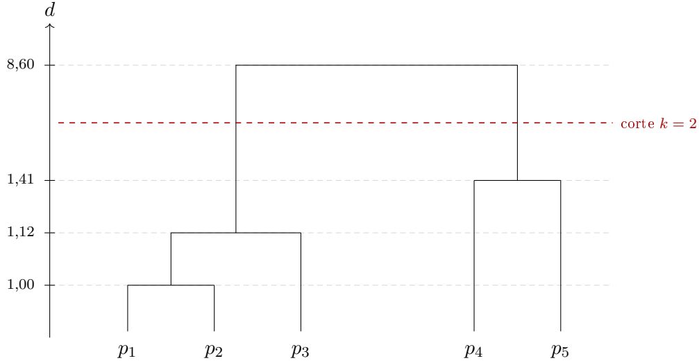
Figura 4: Dendrograma con enlace simple ( escala vertical no proporcional; los valores de d son los reales ). El corte en el intervalo (1,41; 8,60) produce exactamente dos clusters: \{p_1, p_2, p_3\} y \{p_4, p_5\} .
