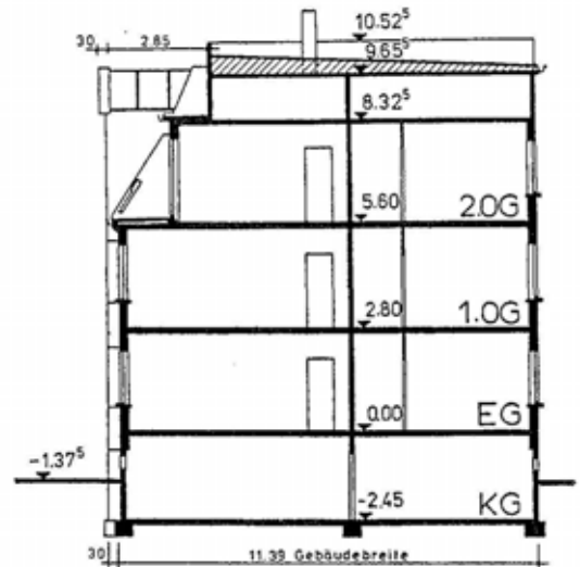
Bild 3.1.2 Ansichten vom Segment 2 (Potsdam) und Gebäudequerschnitt
