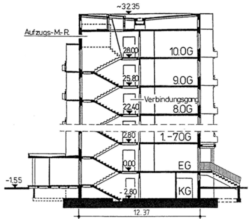
Gebäudequerschnitt (Kellergeschoß + 11 Wohngeschosse)
