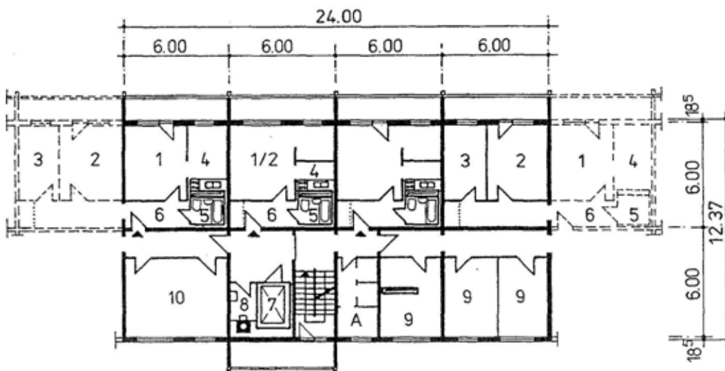
Mittelsegment, Verteilerganggeschoß (8. OG)
