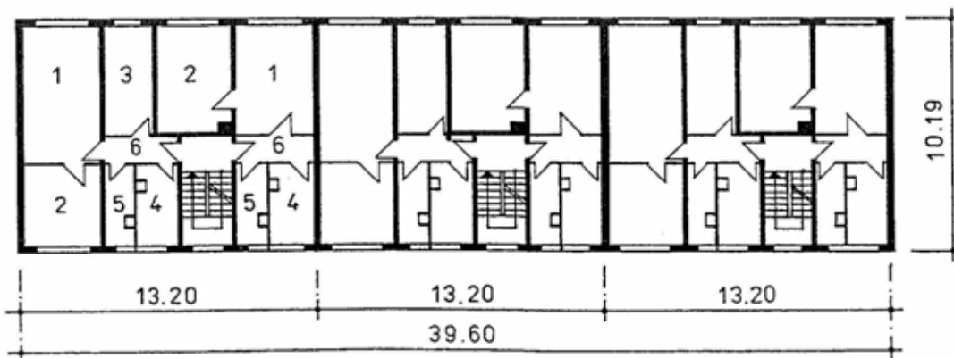
Bild 4.1.1 Grundrisse der Segmente 2 mit Ofen- oder Zentralheizung und Grundriß vom Wohnblock (3 Segmente 2)
