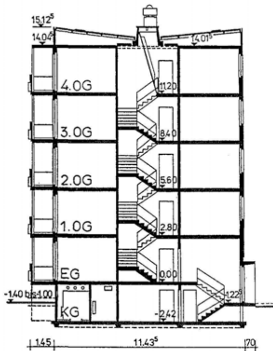
Querschnitt, Mittelsegment IW 76/P2 Halle
