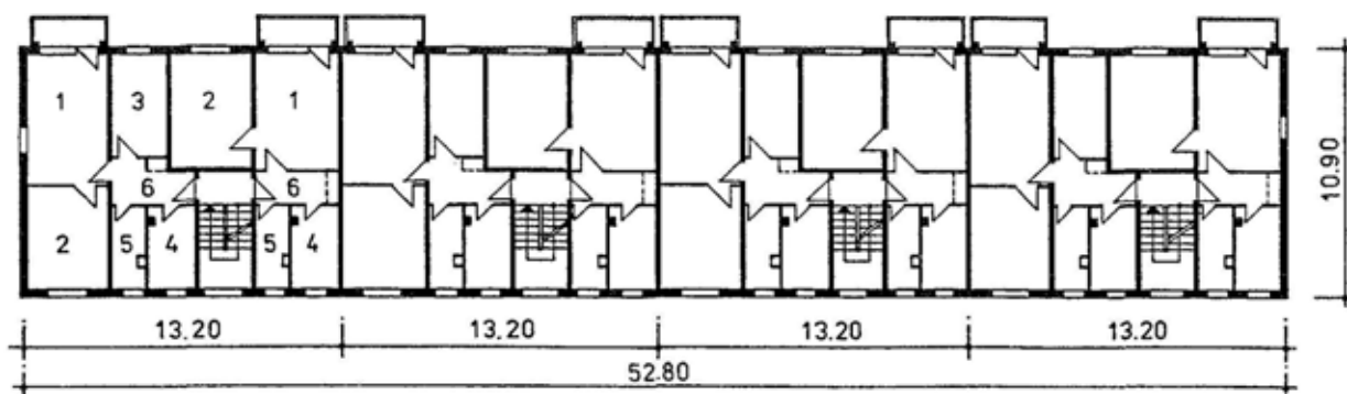
Bild 5.1.1 Grundrisse der Segmente A/B und vom Wohnblock A 44 (4 Segmente A) sowie Gebäudequerschnitt (Segment B)
