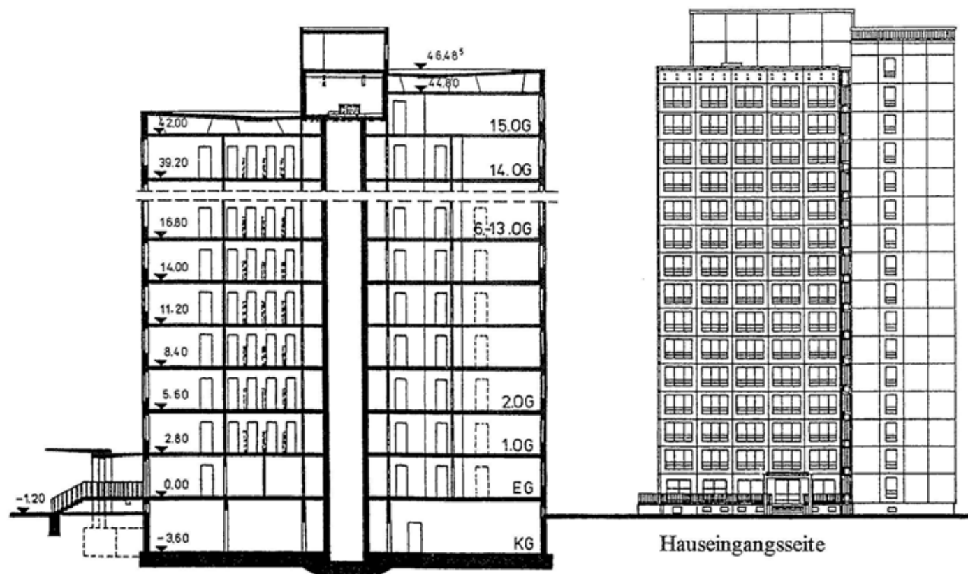
Bild 5.5.3 Grundriß, Schnitt und Ansicht vom Wohnhochhaus PH 16 Leipzig
