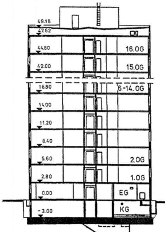
Bild 5.5.2 Grundriß, Schnitt und Ansicht vom Wohnhochhaus WHH 17 Dresden
