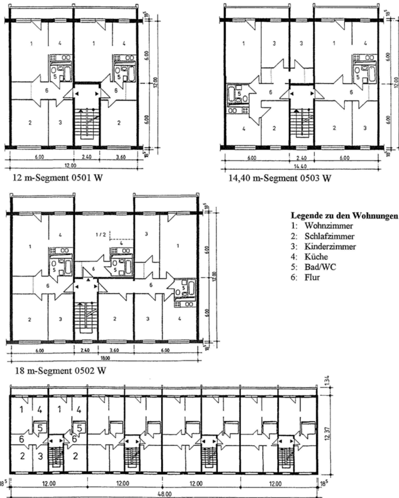
Bild 6.1.1 Grundrisse der Basis-Segmente und des Wohngebäudes MEL B0509 (Anwendung WBK Magdeburg)
