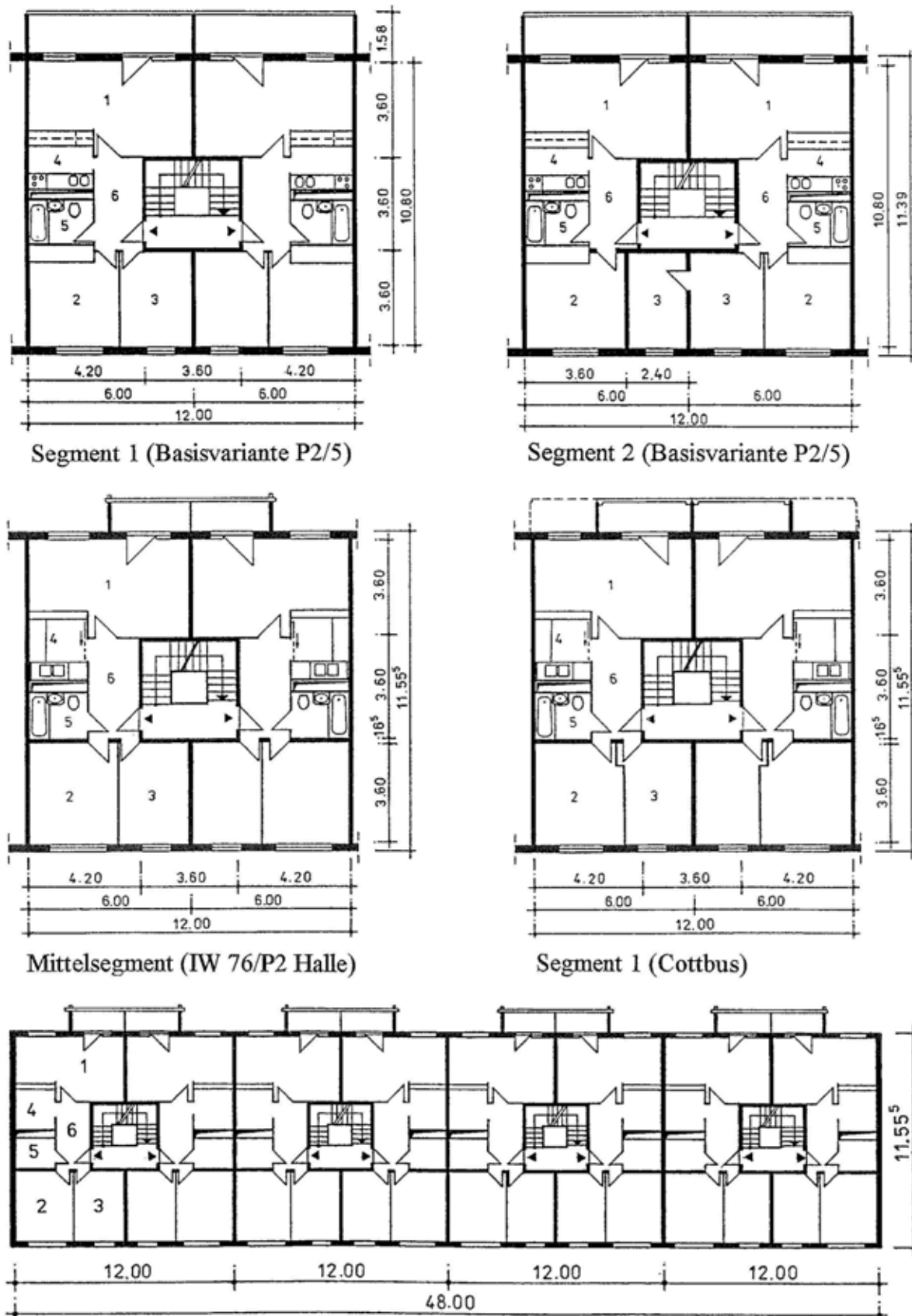
Bild 5.3.1 Grundrisse der Segmente 1, 2 und des Mittelsegmentes / 5geschossig sowie Grundriß vom Wohngebäude (4 Segmente, IW 76/P2 Halle)
