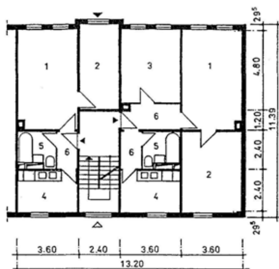
Typ Potsdam: Segment 2
