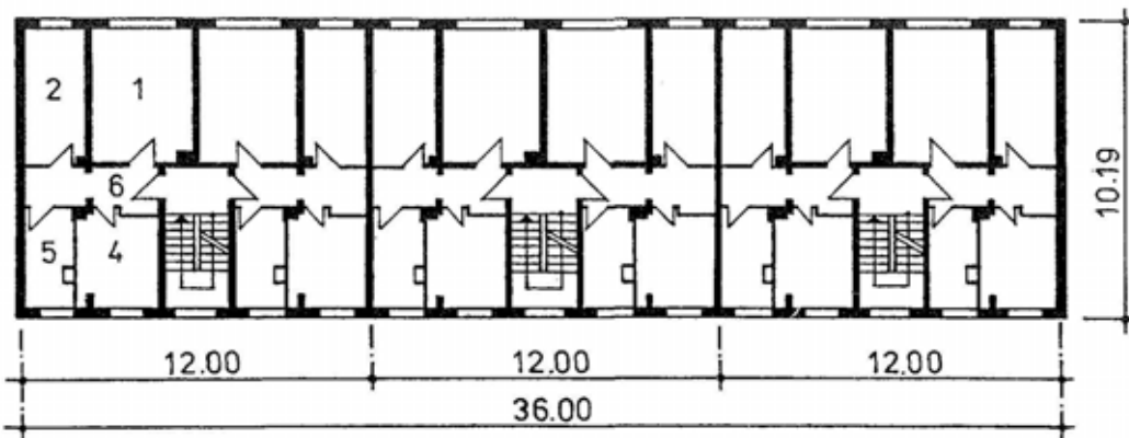
Bild 2.4.1 Grundrisse der Segmente 1 und 2 sowie der Wohnblockzusammenstellung ...33
