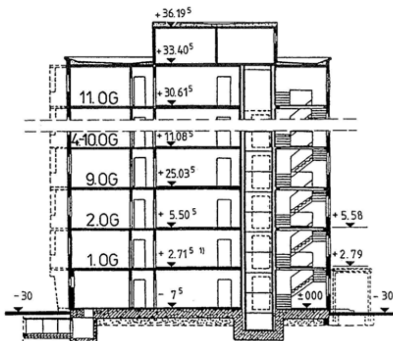
Bild 6.3.1 Grundriß und Schnitt vom Punkthaus PH 12 G
