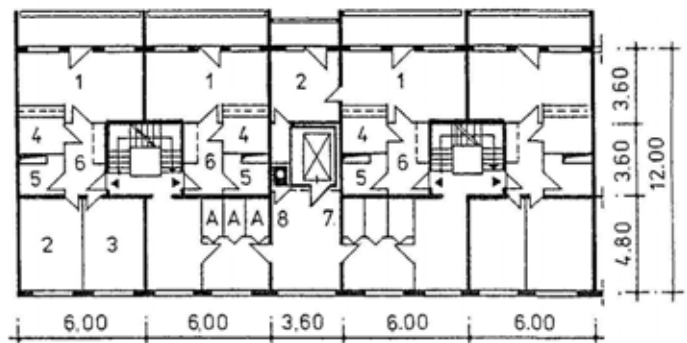
Verteilerganggeschoß Grundrisse, Mittelsegment / 11geschossig, IW 70/P2 Berlin
