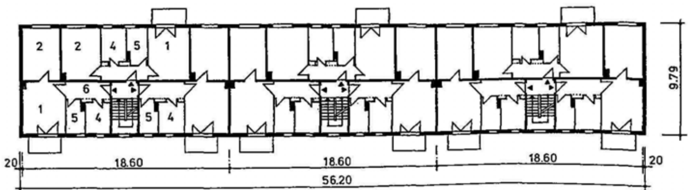
Bild 2.1.1 Grundrisse der Segmente A - C und des Wohnblockes A 43 (3 Segmente A)
