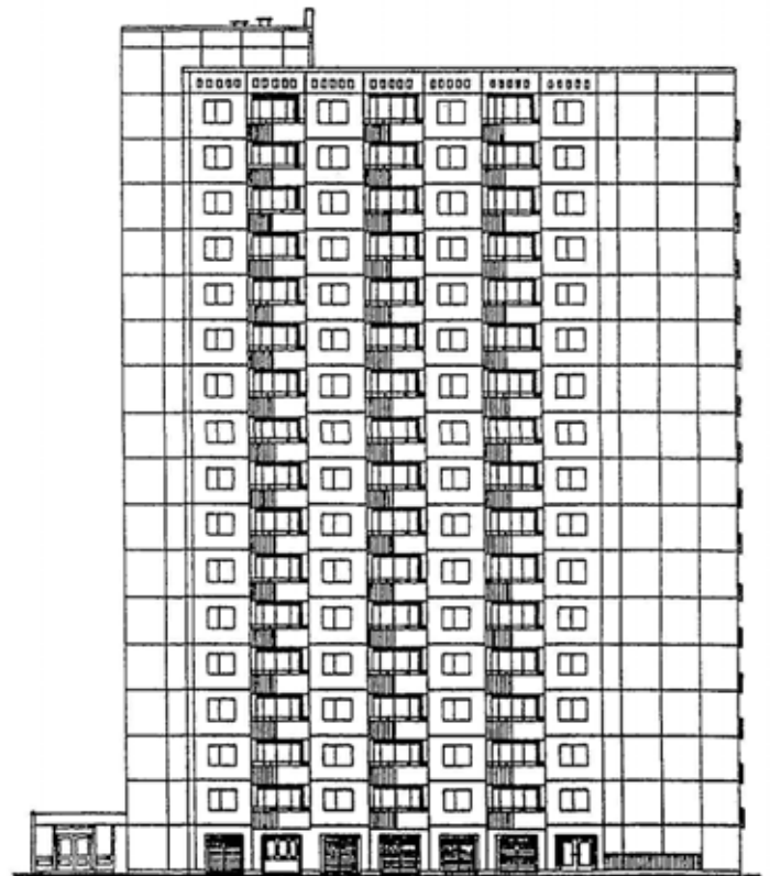
Bild 5.5.2 Grundriß, Schnitt und Ansicht vom Wohnhochhaus WHH 17 Dresden
