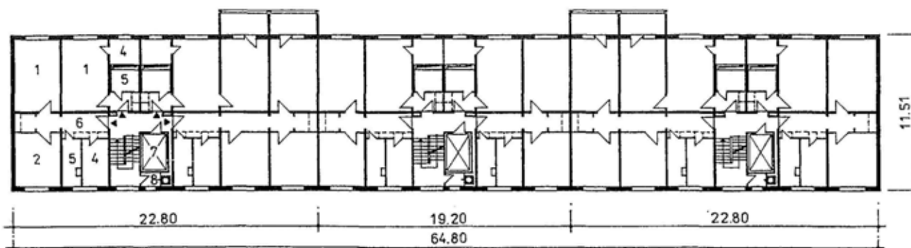
Wohnblock A 103 (1. - 8. OG)
