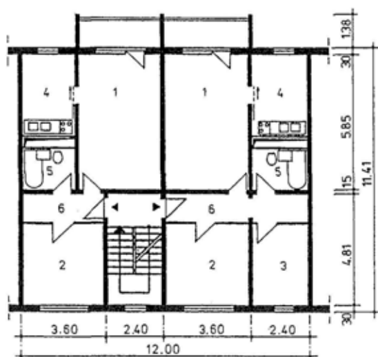
Typ Hagenow: Segment 2
