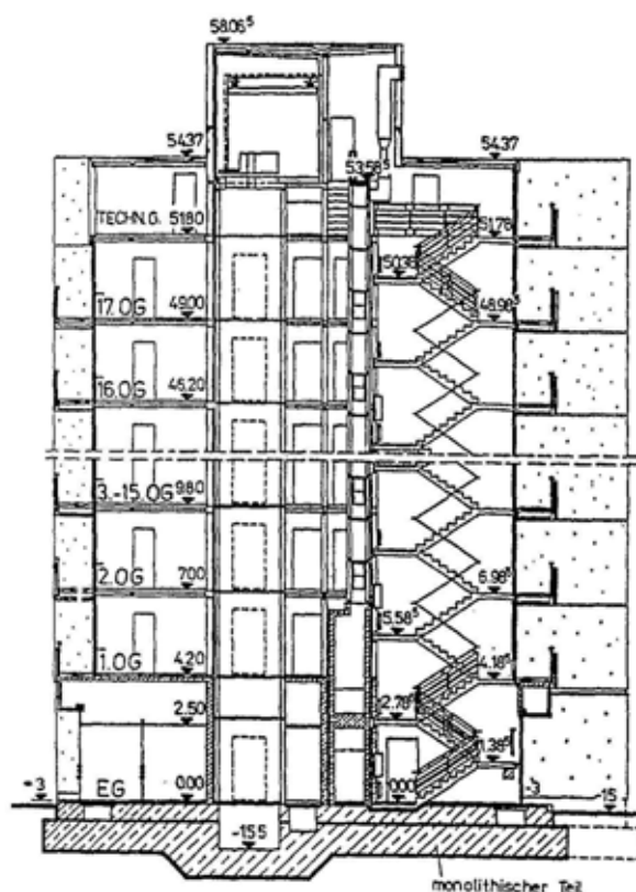
Bild 6.4.1 Grundriß und Schnitt vom Wohnhochhaus WHH GT 18
