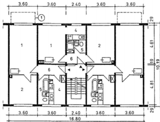
Segment 1 (Ofenheizung, WW/Gas)
