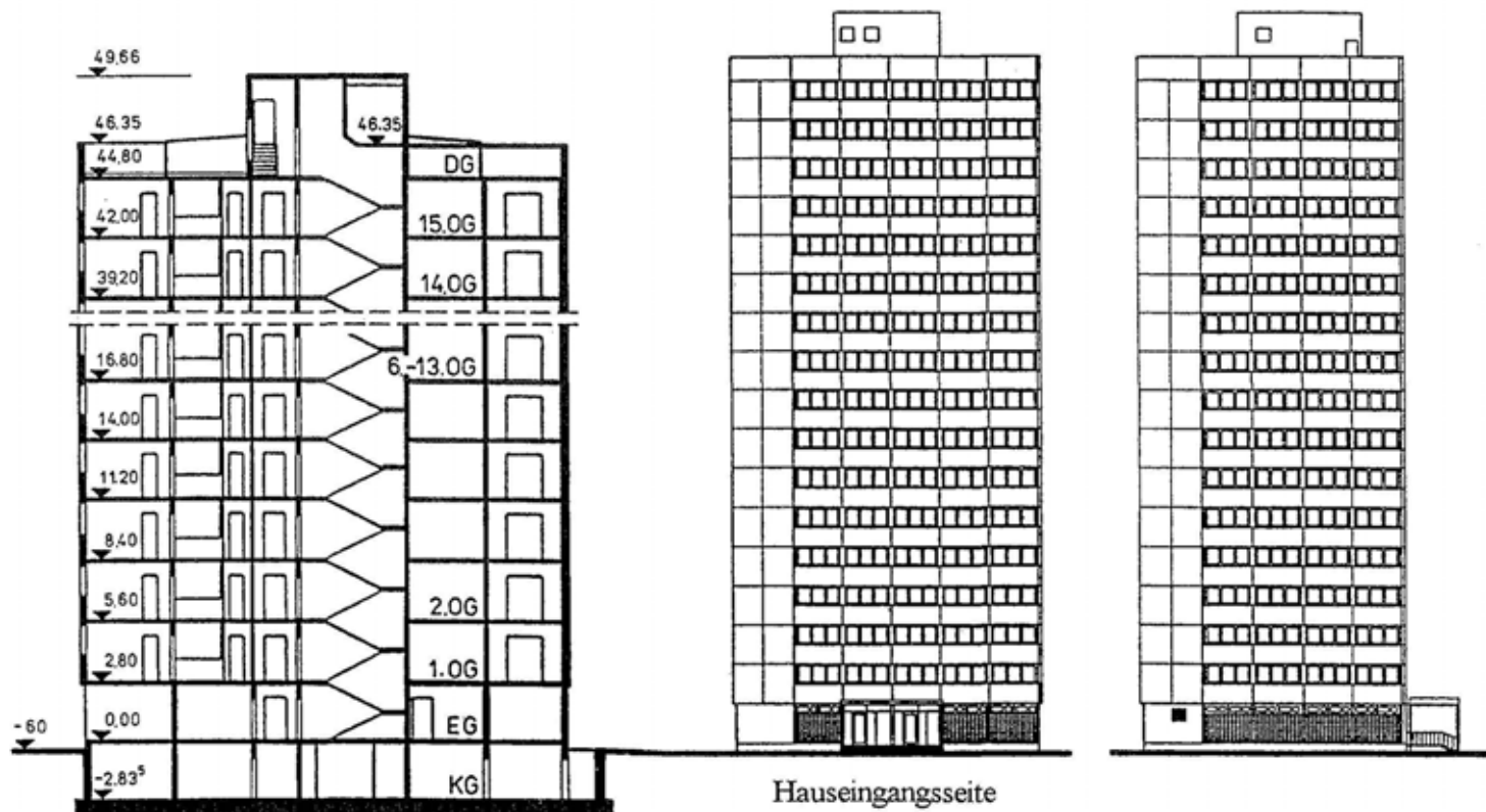
Bild 5.5.1 Grundriß, Schnitt und Ansichten vom Wohnhochhaus PHH 16 Frankfurt/Oder
