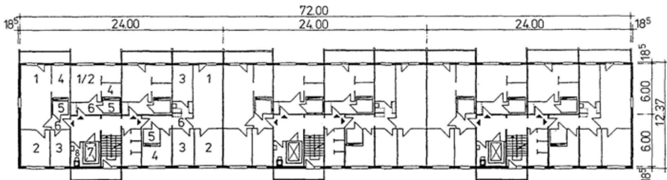
Mittelsegment, Verteilerganggeschoß (8. OG)
