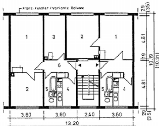
Segment 2 (Ofenheizung WW/Gas)
