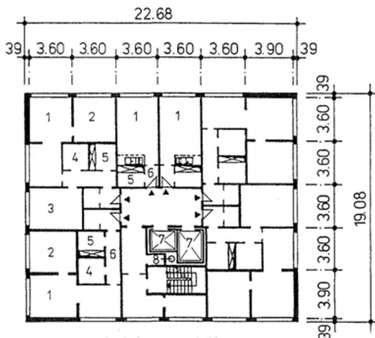
Normalgeschoß (1. - 15. OG)
