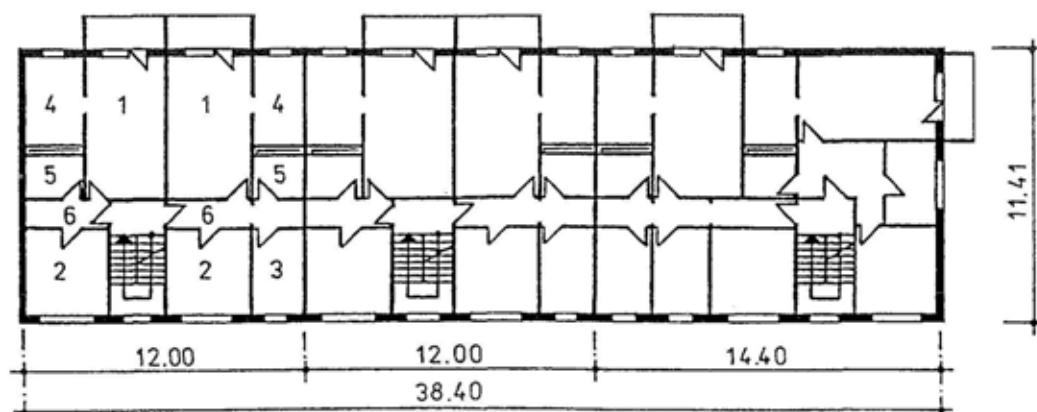
Bild 3.1.1 Grundrisse der Segmente 1 - 3 (Typen Potsdam und Hagenow) und vom Wohngebäude Typ Hagenow
