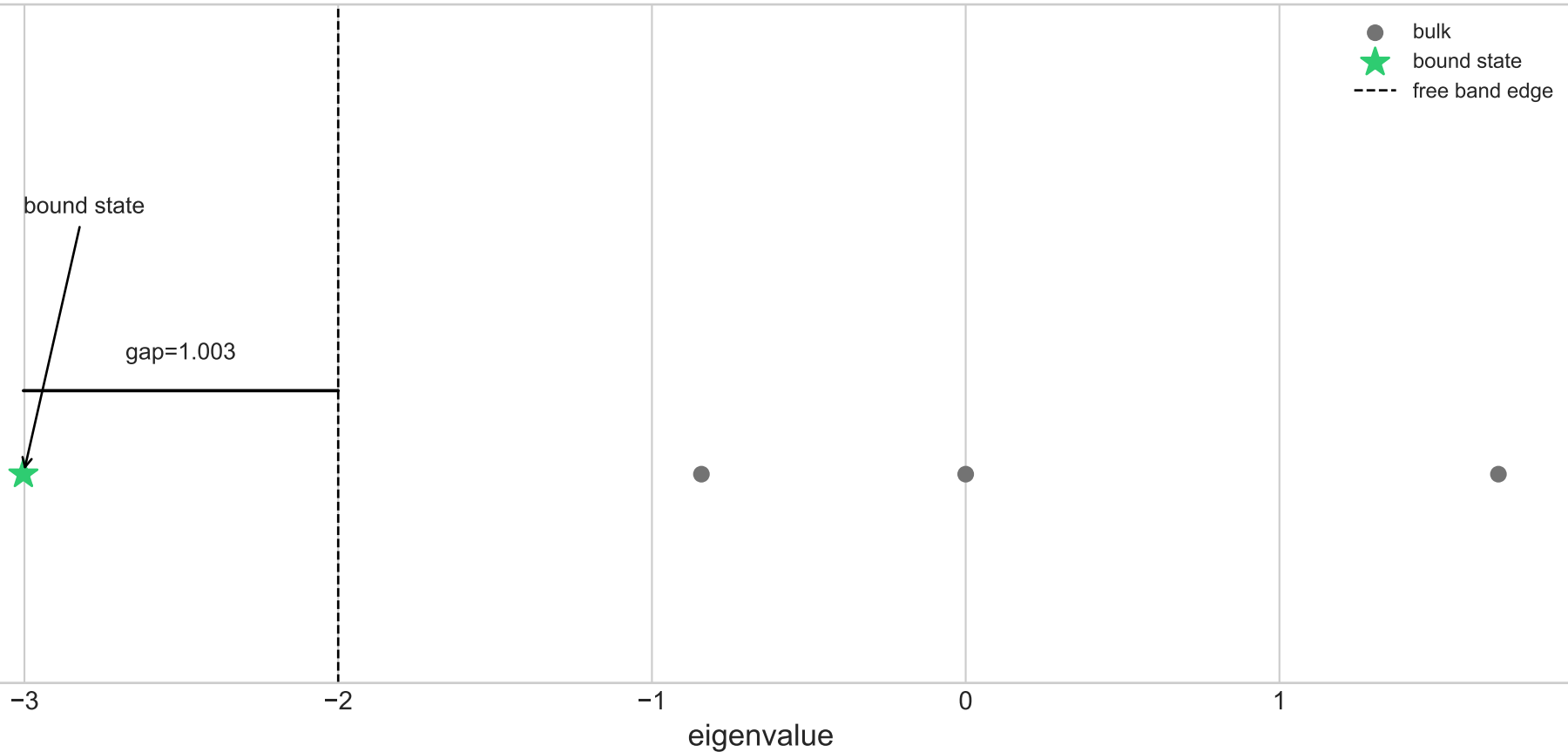
Eigenvalue spectrum — 06_2d_tiny_corner_block
