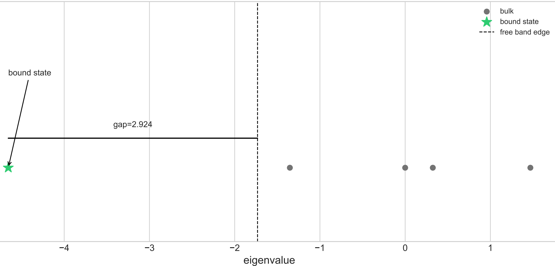
Eigenvalue spectrum — 01_1d_tiny_single_gap
