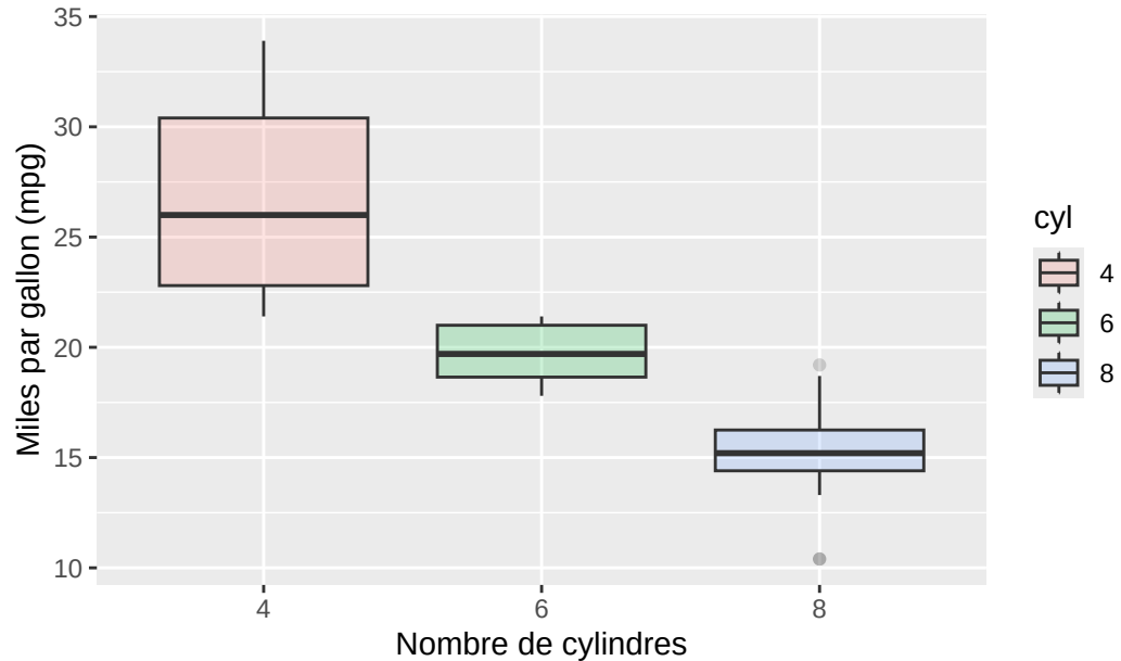
Miles par gallon (mpg) selon le nombre de cylindres dans mtcars
