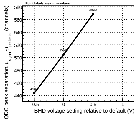
BHD paddle 06
