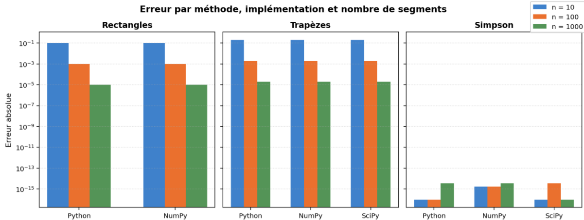
Figure 3 — Erreur absolue pour n = 10, 100 et 1000 . L'échelle log permet de comparer les 3 groupes. Simpson est exact indépendamment de n et de l'implémentation. Pour rectangles et trapèzes, l'erreur diminue d'un facteur 100 quand n est multiplié par 10 (cohérent avec O(h^2) ).
