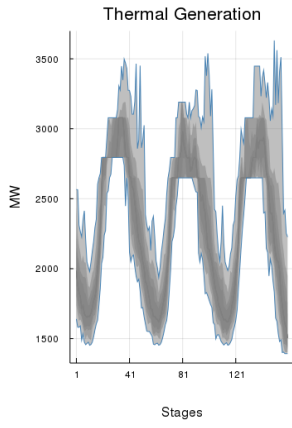
Fig. 2. Thermal Generation
