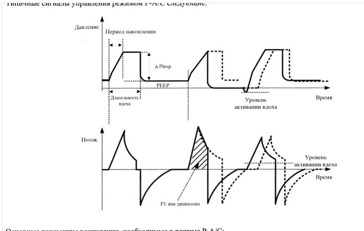
Рис. 1. Кривые давления и потока в режиме P-A/C. Давление нарастает за время Tslope до уровня \Delta P_{\text{insp}} над PEEP и удерживается до конца вдоха; инспираторный поток убывает по мере выравнивания давления. Пунктиром показан цикл, запущенный инспираторной попыткой пациента.
