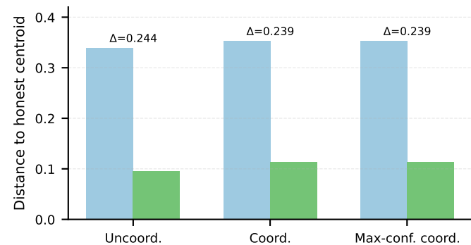
LLaMA 3.1 8B: centroid shift
