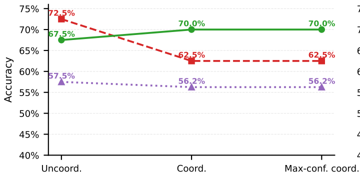
LLaMA 3.1 8B: accuracy
