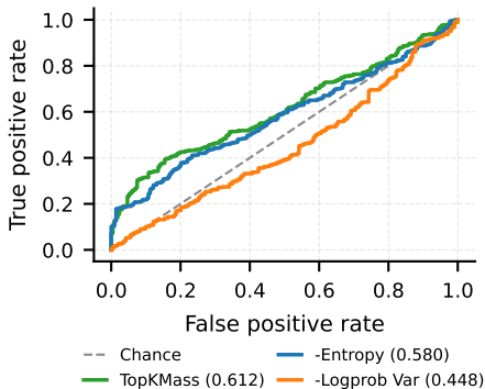
ROC
