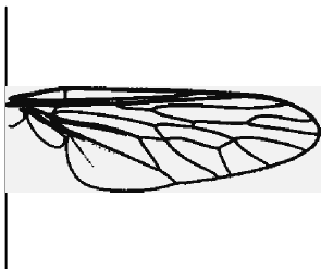
Asilidae wing
