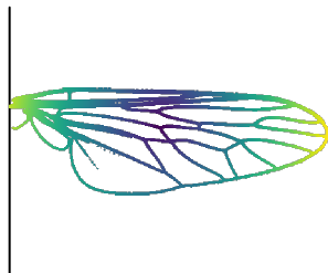
A-11 radial
