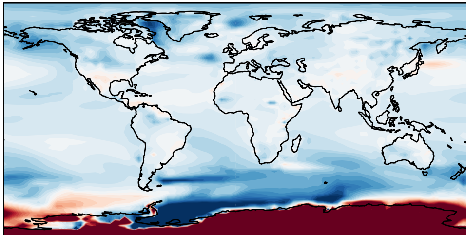
TEMPERATURE AT 1.5M: xogzl - xoorb
