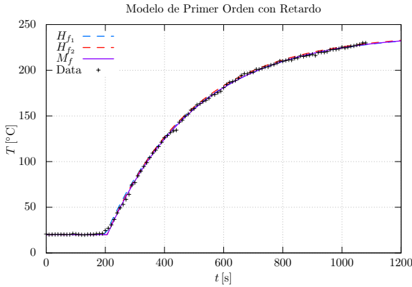
Figura 2. Modelos de primer orden con retardo.
