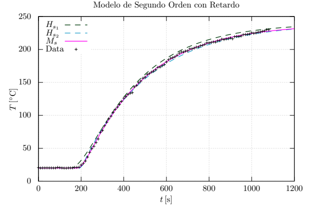
Figura 3. Modelos de segundo orden con retardo.
