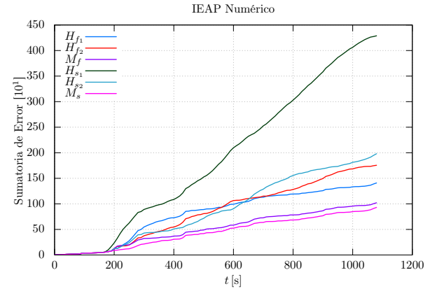
Figura 4. Integral del Error Absoluto de Predicción.
