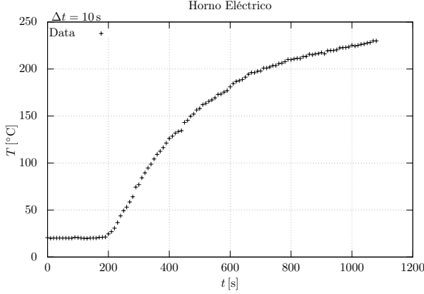
Figura 1. Temperaturas registradas.
