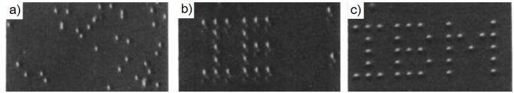
Figura 3: Manipulación de la punta de STM comenzando con a) muestra de xenón dosificada aleatoriamente, b) en construcción - mover el átomo de xenón a la posición deseada, y c) realización de la manipulación.
