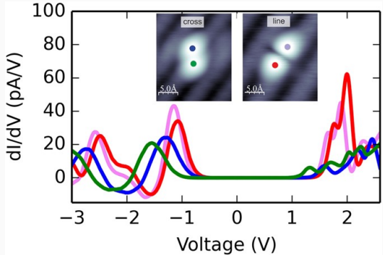
Figura 9: Conductancia diferencial experimental ( dI/dV ). Los picos se correlacionan con las bandas calculadas en DFT.
