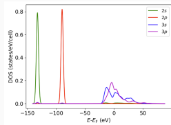
Figura 7: LDOS Teórica: Contribución espacial y de estados profundos.
