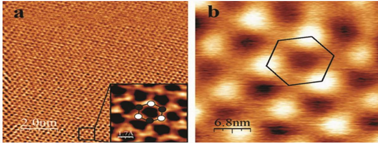
Figura 4: Imágenes STM de HOPG: (a) Superficie normal con resolución atómica (0.246 nm entre puntos). Los puntos claros indican átomos de carbono sin un átomo en la capa inferior directa, mientras que los oscuros sí lo tienen. (b) Súperred que muestra un patrón hexagonal periódico, originado por un desajuste espacial entre la capa superficial y la inferior. Obtenidas con un equipo JEOL JSPM-5200 (resolución replicable con Nanosurf E-STM).
