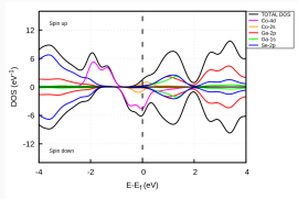
Figura 8: PDOS Teórico (QE): Proyección por orbitales.
