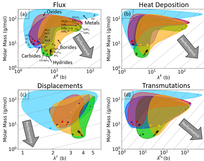
Figura 6: Materiales para blindaje de masa mínima, protegiendo Si de un espectro de fisión rápido. [8]
