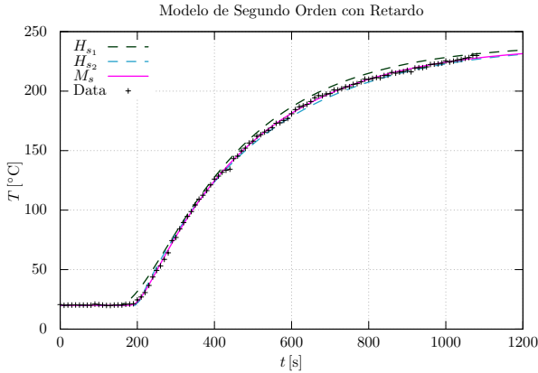
Figura 4. Modelos de segundo orden con retardo.
