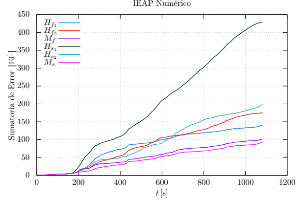
Figura 5. Integral del Error Absoluto de Predicción.
