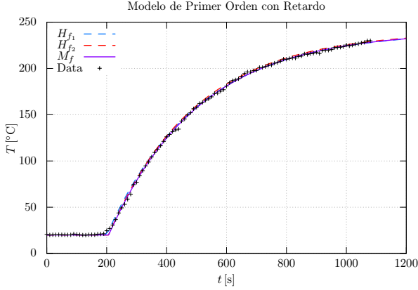
Figura 3. Modelos de primer orden con retardo.
