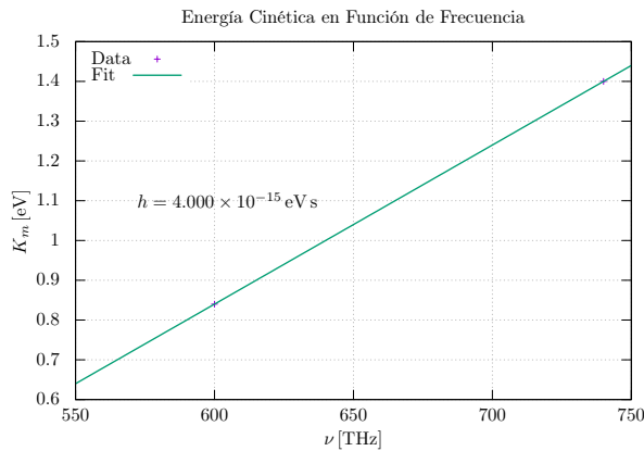
Figura 4. Energía cinética de los electrones en función de la frecuencia.
