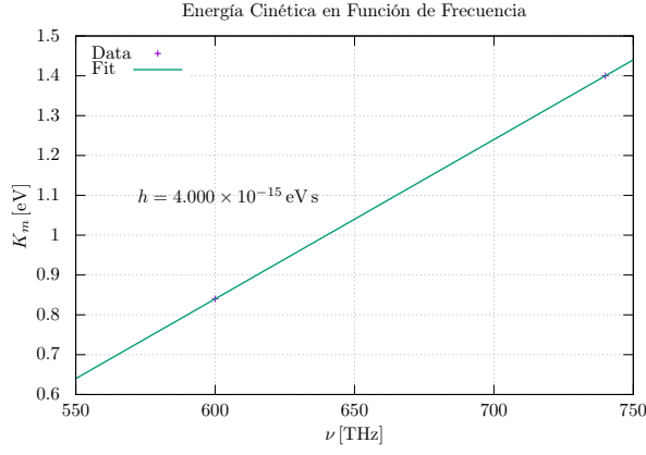
Figura 3. Energía cinética de los electrones en función de la frecuencia.
