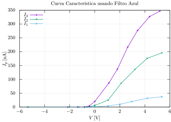
Figura 1. Curva característica de la fotocelda con filtro azul.
