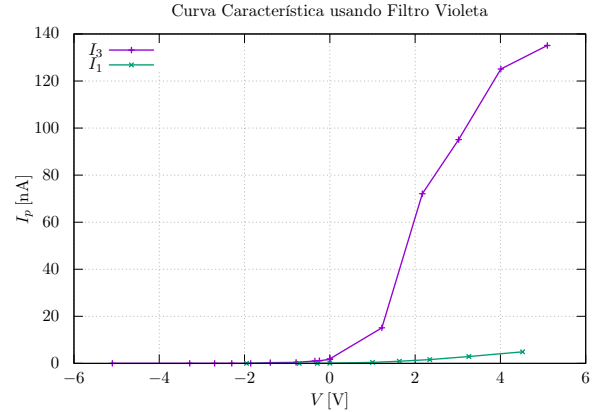
Figura 2. Curva característica de la fotocelda con filtro violeta.
