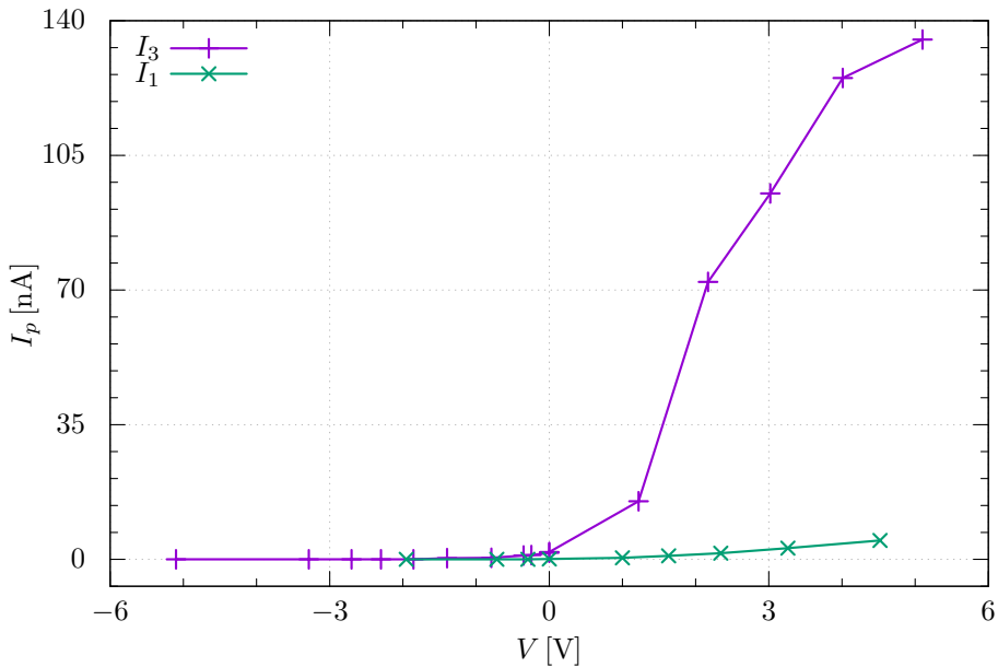
Curva Característica usando Filtro Ultravioleta
