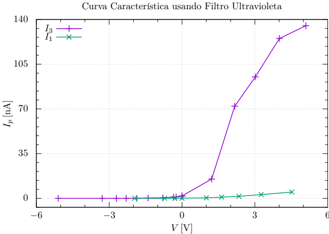
Figura 3. Curva característica de la fotocelda con filtro ultravioleta.
