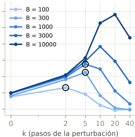
Bajada estocástica + reinicios
