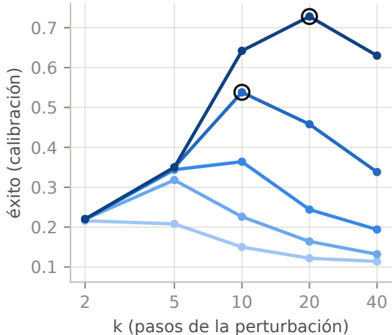
Bajada simple + reinicios
